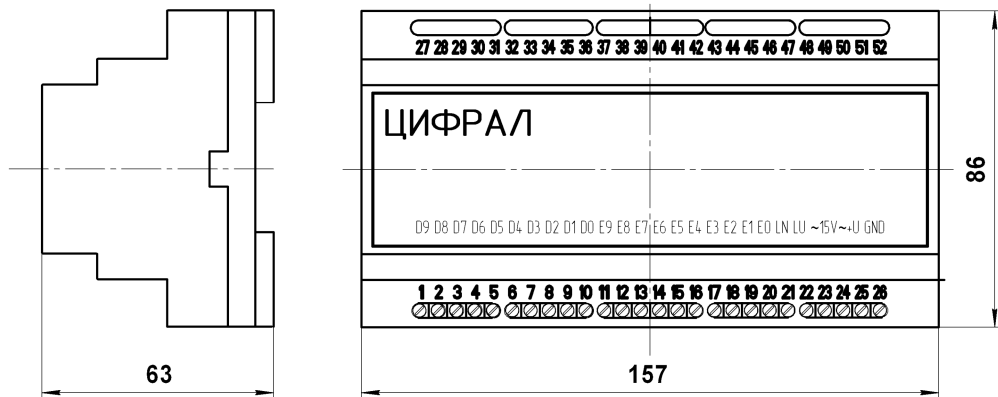
Рисунок В.2 Габаритные и установочные размеры коммутатора КИФРАЛ КМГ-100.1
