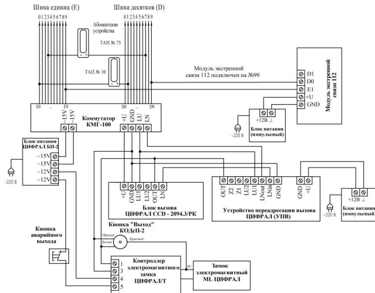
Рисунок Г.4 - Схема подключения блока вызова с устройством передиресации вызова и модулем экстренной связи 112
