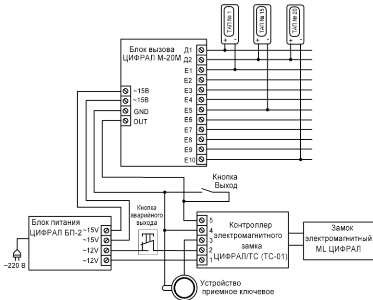
Рисунок Б.2 Схема подключения домофона ЦИФРАЛ М-20М
