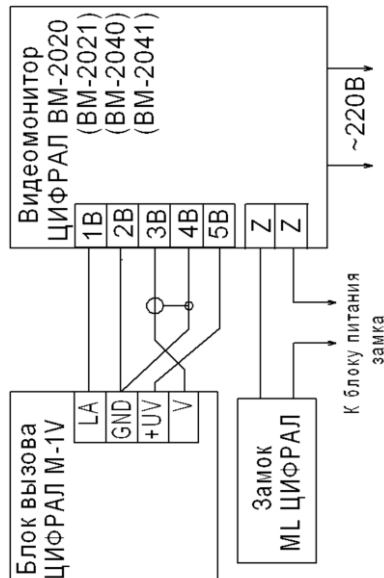
Схема подключения блока вызова
