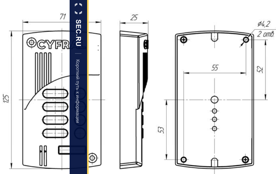
Рисунок А.2 Установочные и габаритные размеры блока вызова ЦИФРАЛ М-4.1М (ЦИФРАЛ М-4.1М/V, ЦИФРАЛ М-4.1М/VC)
