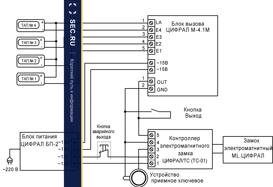
Рисунок Б.3 Схема подключения домофона ЦИФРАЛ М-4.1М
