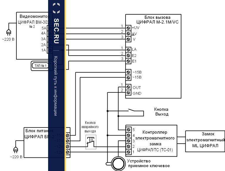
Рисунок Б.2 Схема подключения домофона ЦИФРАЛ М-2.1М/ТС
