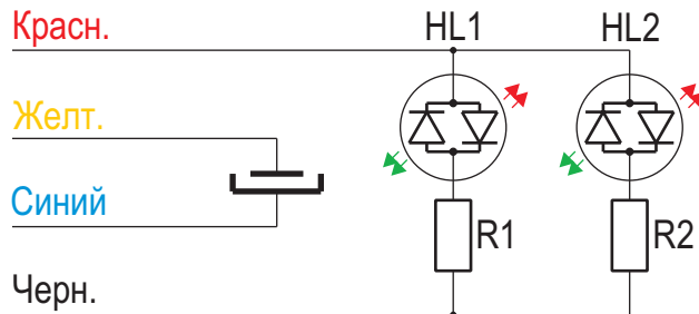
Рис. 2 Электрическая схема
