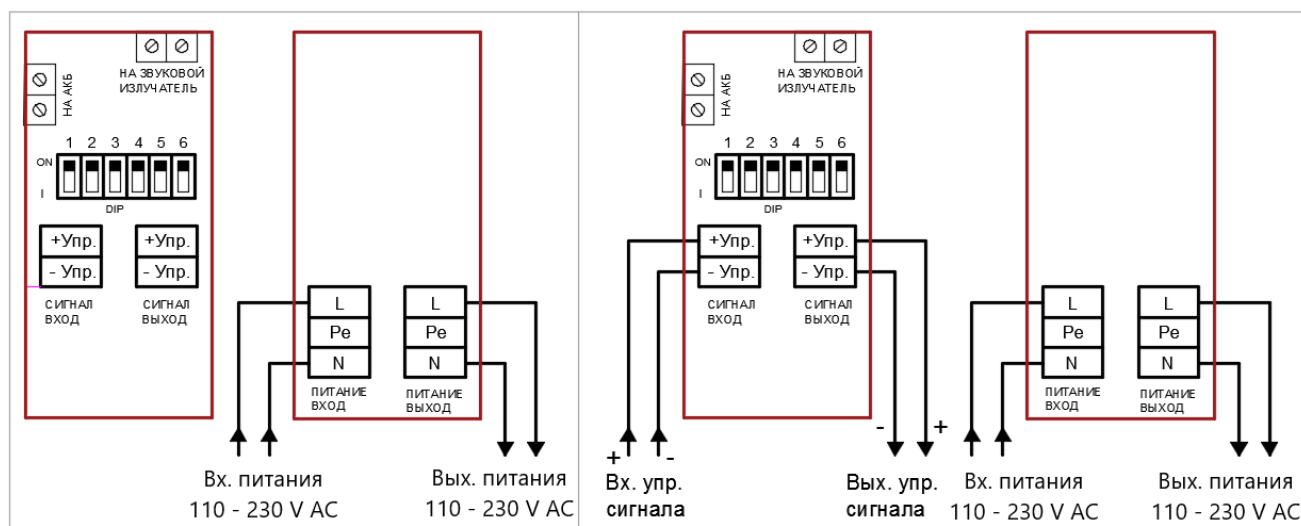
Рисунок 7 – Схема 2-х и 4-х проводного подключения ТС3В-Exd-A/H-Прометей 220В. Номинал управляющего сигнала: 12÷36В DC, 12÷28В AC.
