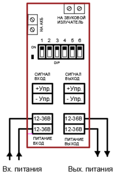
Рисунок 3 – Схема 2-х проводного подключения оповещателя пожарного взрывозащищенного ТСВ 12÷36В. Номинал управляющего сигнала: 12÷36В DC, 12÷28В AC.
