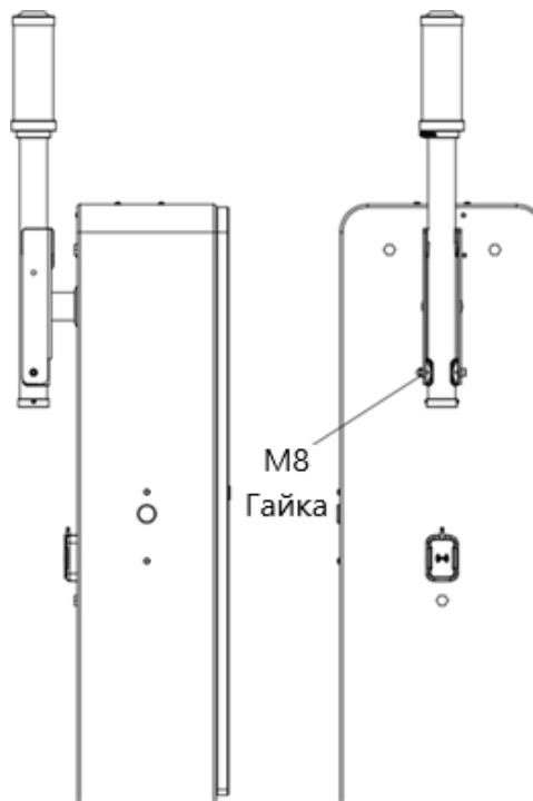
Рисунок 2.14 Фиксация стрелы
