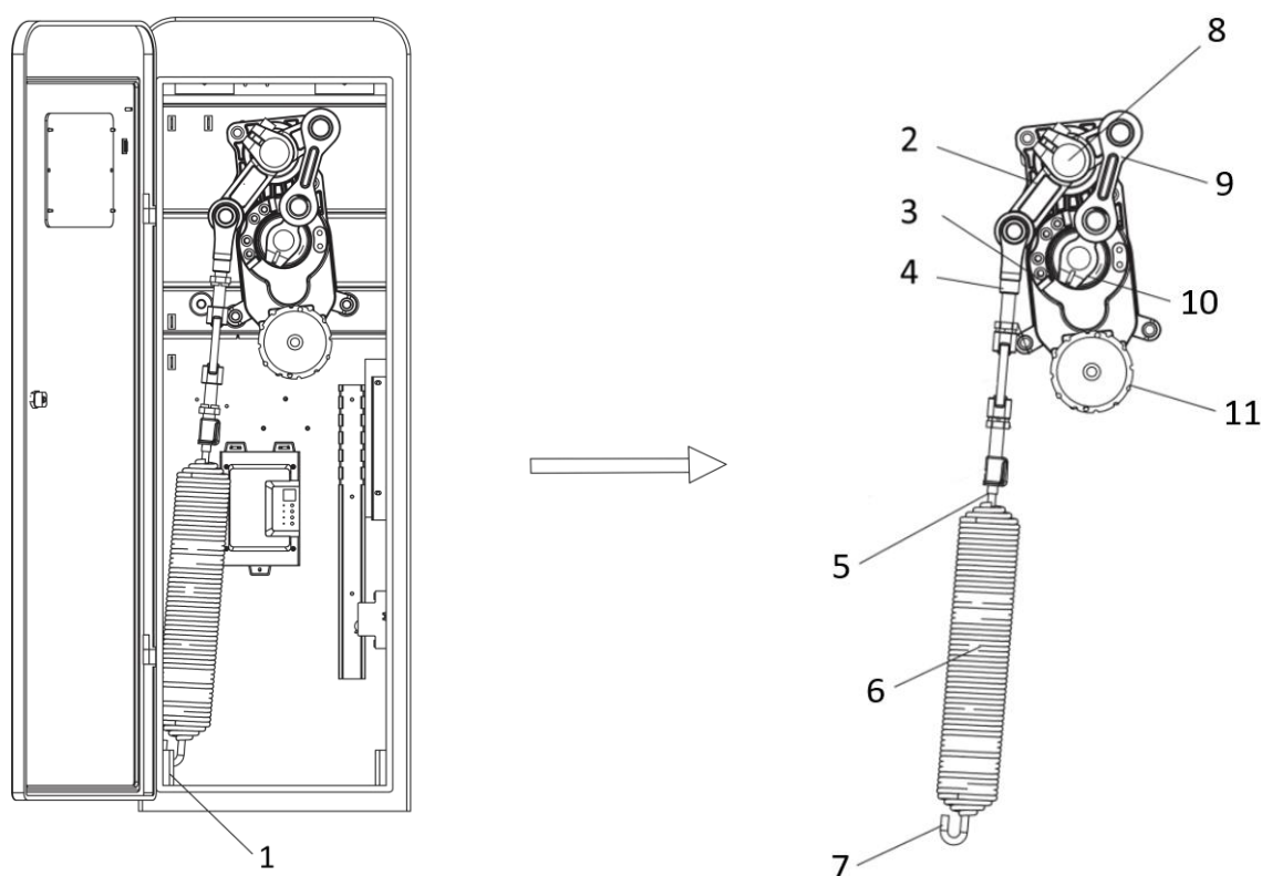
Рисунок 1.2 Внутренняя конструкция
