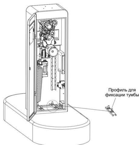
Рисунок 2.4 Фиксация тумбы
