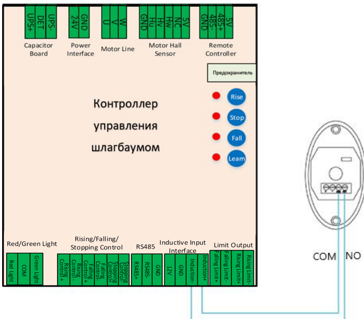
Рисунок 2.34 Подключение к активному инфракрасному датчику движения
