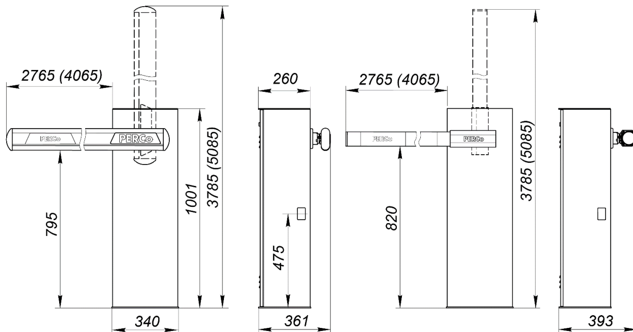
Рисунок 1. Габаритные размеры шлагдаума
