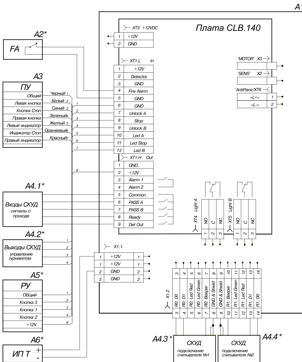
Схема соединений турникета TB01.9A и дополнительного оборудования
