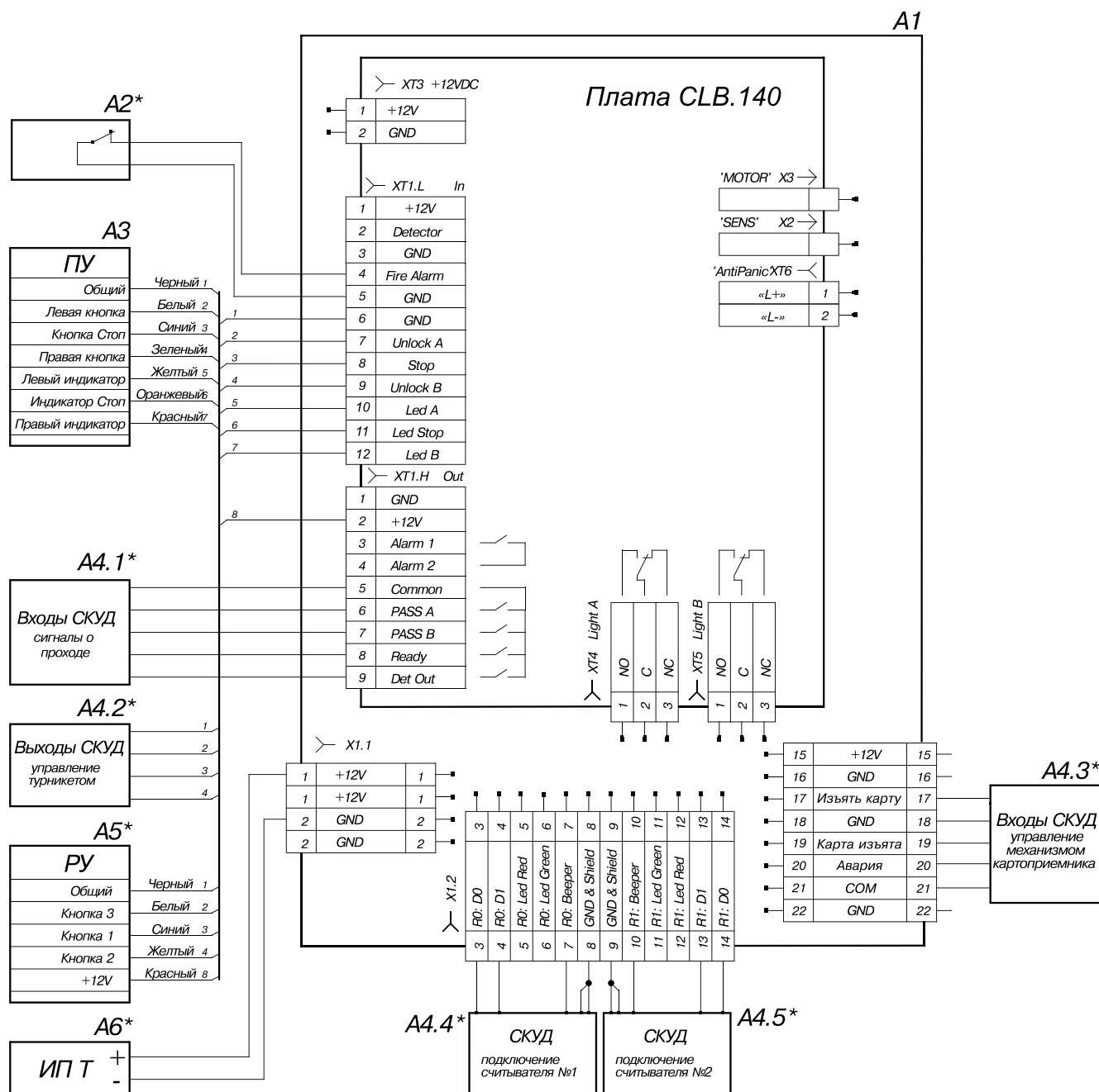
Схема соединений турникета TBC01.9A и дополнительного оборудования
