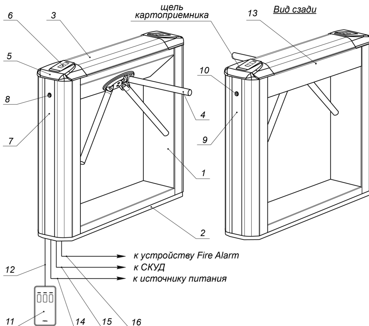
Рисунок 2. Устройство турникета
