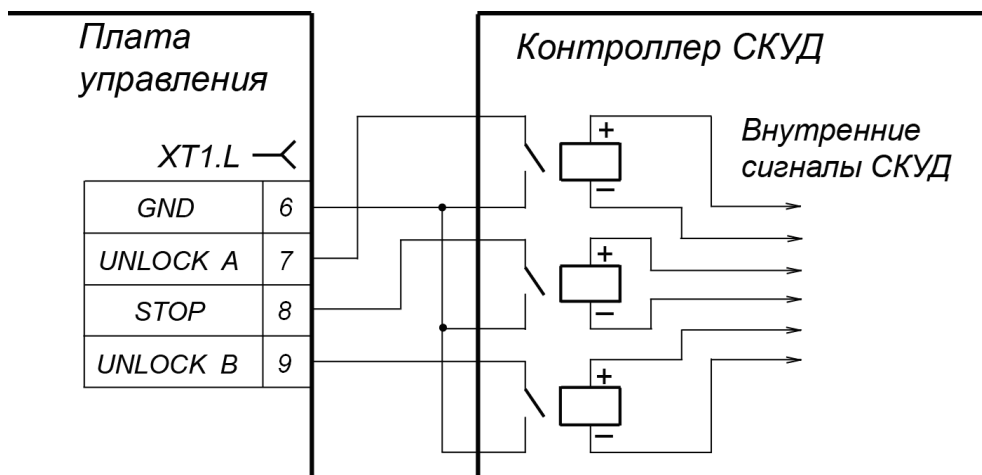
Рисунок 6. Управляющие элементы – нормально разомкнутый контакт реле
