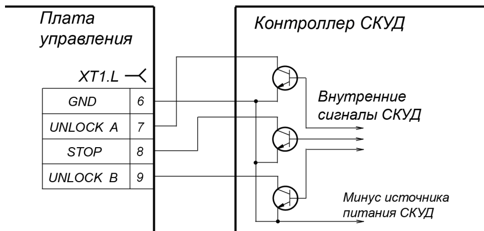
Рисунок 7. Управляющие элементы – схема с открытым коллекторным выходом
