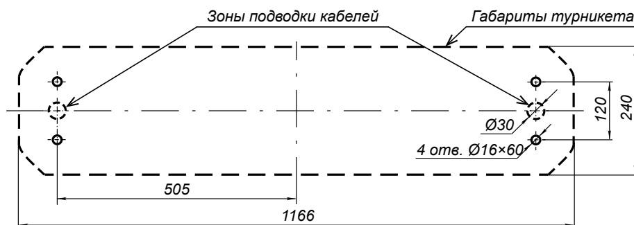
Схема разметки отверстий в полу под крепление стойки турникета и зоны для подвода кабелей
