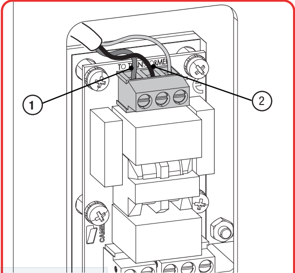
СЕТЕВОЕ ЭЛЕКТРОПИТАНИЕ 230 В ПЕРЕМЕННОГО ТОКА (Заводская настройка)
