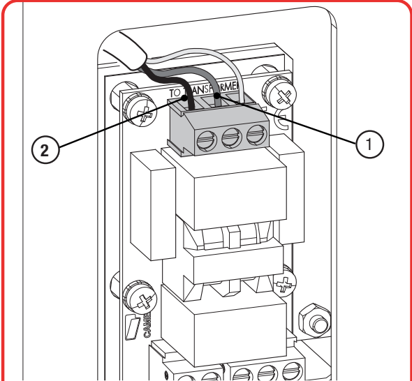
СЕТЕВОЕ ЭЛЕКТРОПИТАНИЕ 120 В ПЕРЕМЕННОГО ТОКА (Поменяйте местами провода 1 и 2, как показано на рисунке)
