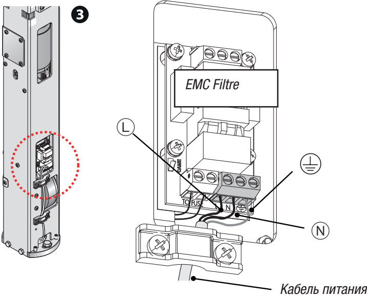
СЕТЕВОЕ ЭЛЕКТРОПИТАНИЕ 230 В ПЕРЕМЕННОГО ТОКА (Заводская настройка)
