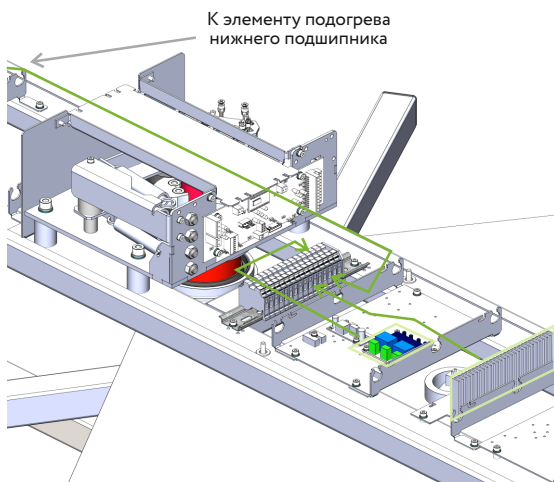
Рисунок 10.3 - Элементы подогрева в корпусе механизма
