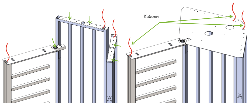
Рисунок 9.8 - Турникет с установленной крышкой зоны прохода Максимально надёжное российское оборудование СКУД · СОТ · ОС · ИСБ
