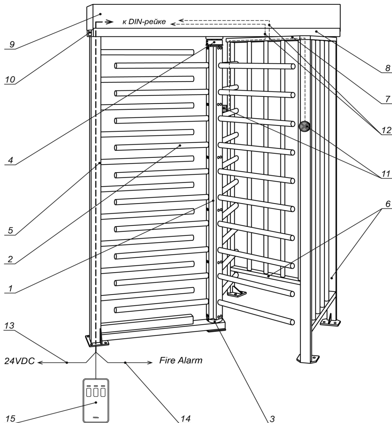
Рисунок 2. Устройство турникета:
