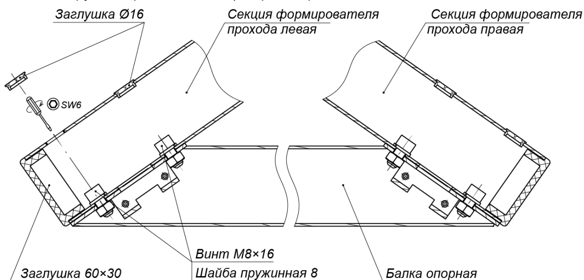
Рисунок 12. Крепление балки опорной (7) к секциям (6) формователя прохода
