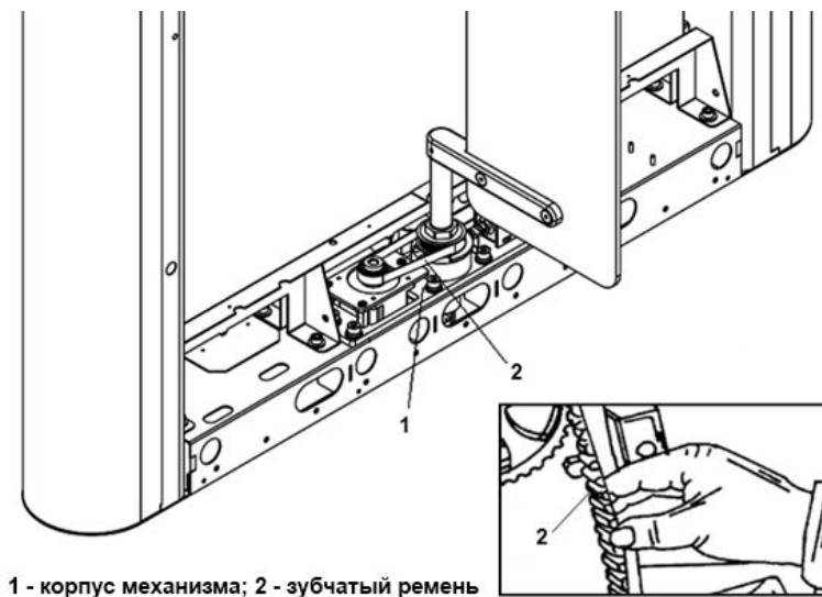
1 - корпус механизма; 2 - зубчатый ремень
