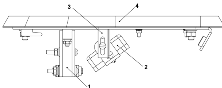
Рисунок 14- Рекомендуемый вариант установки считывателя бесконтактных карт
