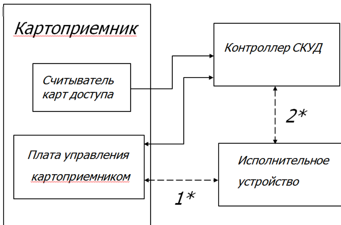
Рисунок 20- Структурная схема №3
