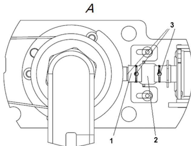
Рисунок 10 – Корпус механизма турникета
