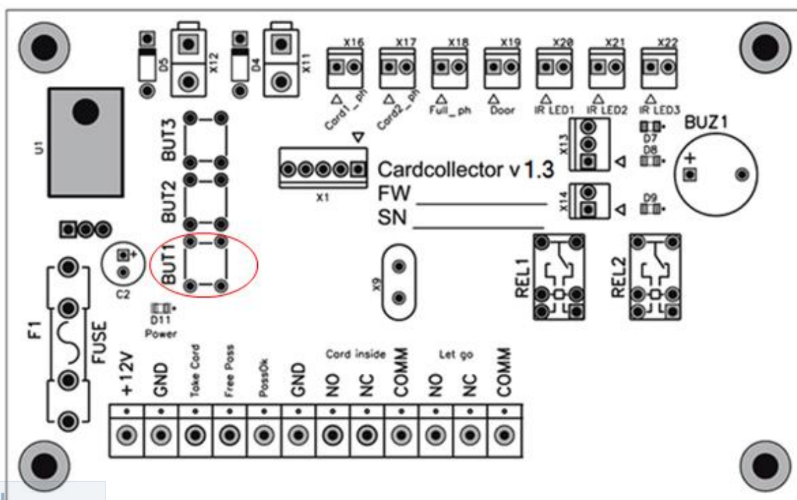
Внешний вид платы картоприемника.
