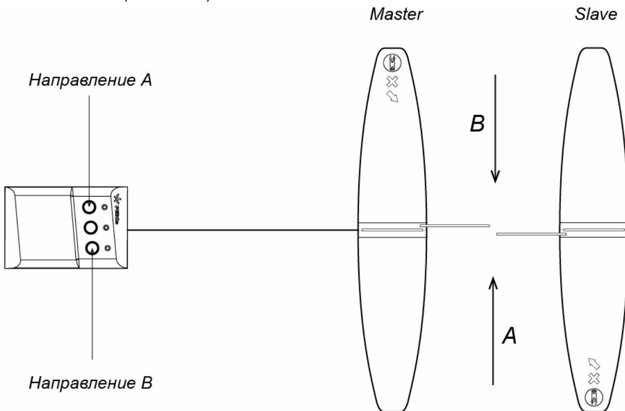
Рисунок 10. Стандартная ориентация ПДУ относительно секций турникета
