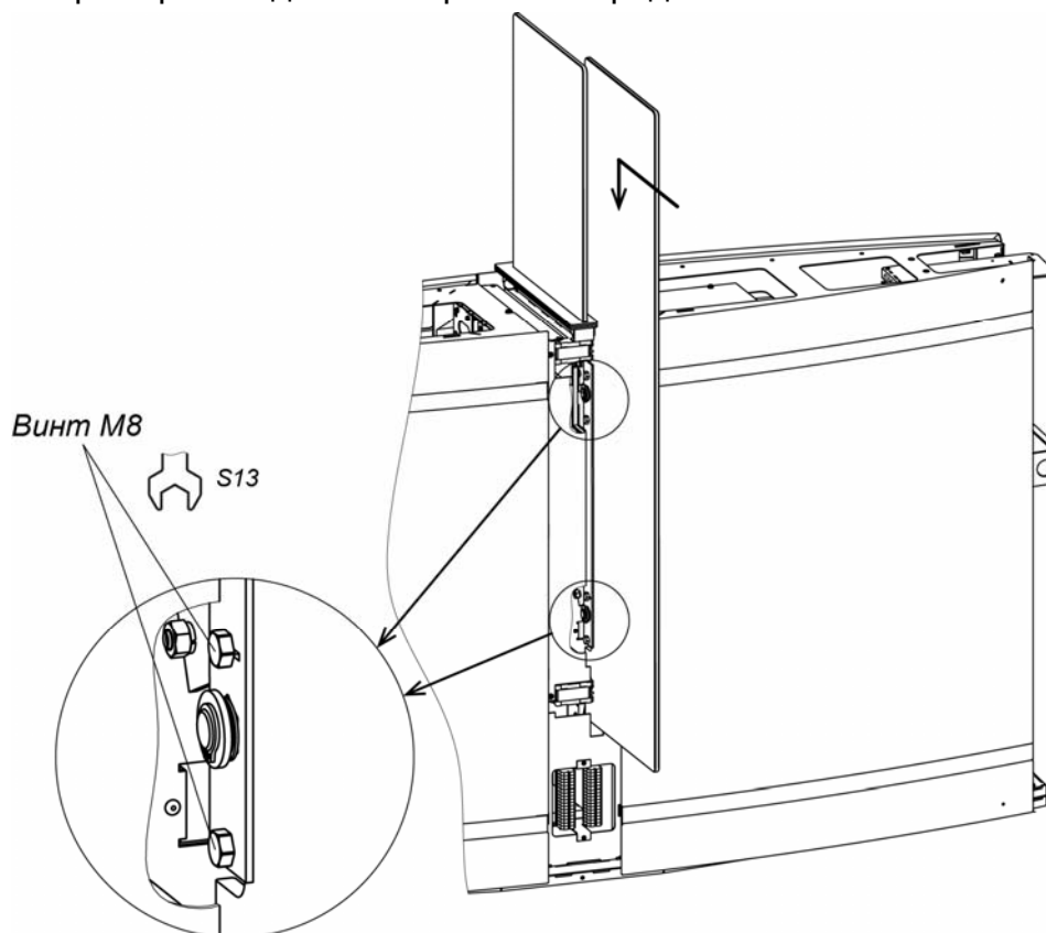
Рисунок 24. Монтаж створки
