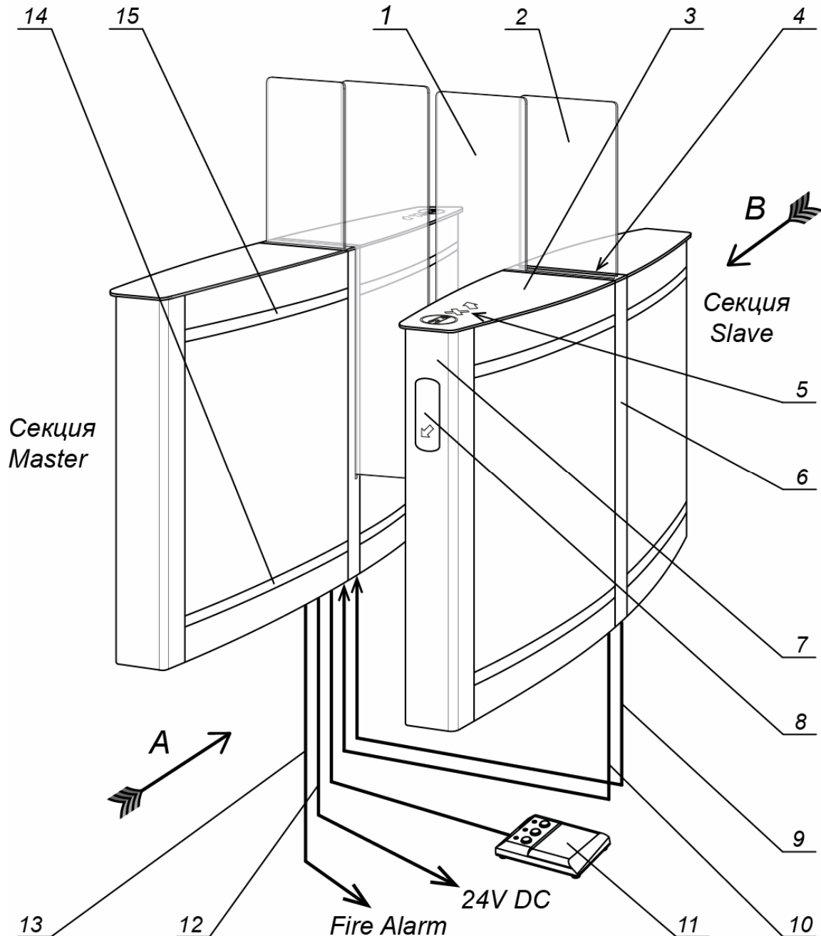
Рисунок 3. Внешний вид и устройство PERCo-ST-02
