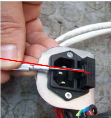
Замена предохранителя
