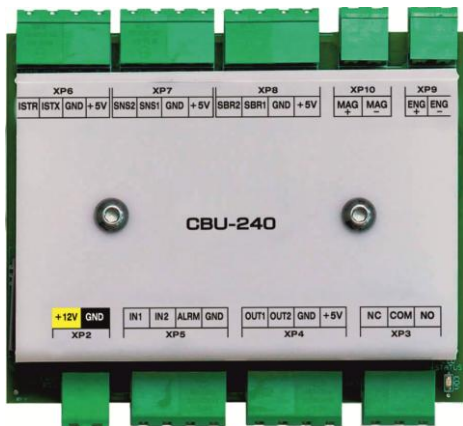
Рисунок 6.3.1 Контроллер управления турникетом «CBU-240»
