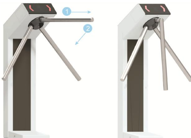
Рисунок 6.5.2 - Принцип работы планок «Антипаника».
