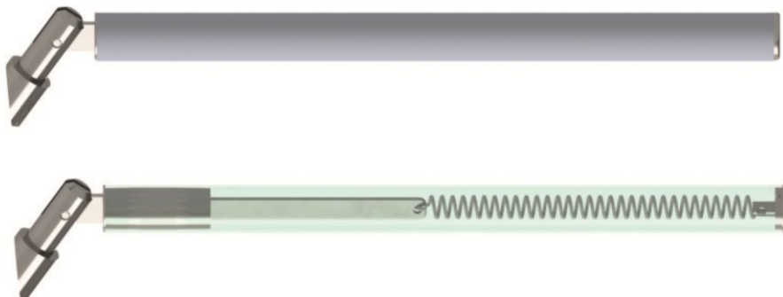
Рисунок 6.5.1 - Преграждающие планки «Антипаника»
