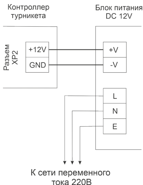
Рисунок 8.4.1 - Подключение питания к турникету
