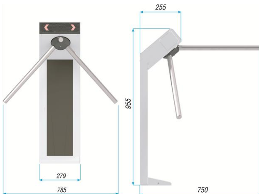
Рисунок 5.1 - Габаритные размеры турникета с планками
