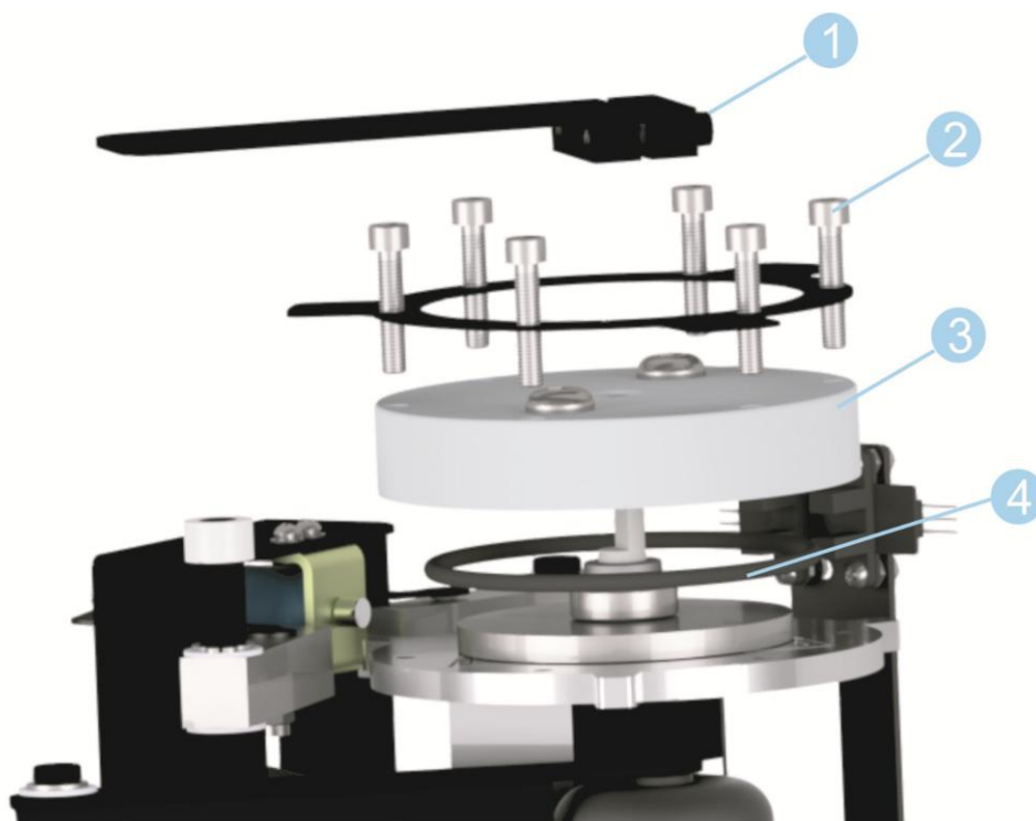
Рисунок 12.3.1 - Порядок замены уплотнительного кольца.
