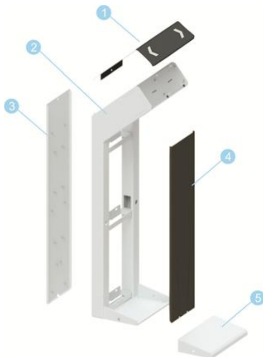
Рисунок 6.1.1. - Элементы корпуса турникета
