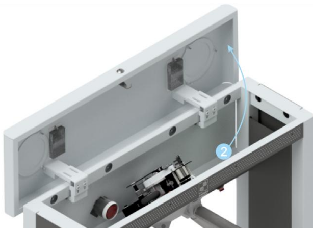
Рисунок 12.1.1 Демонтаж верхней крышки турникета
