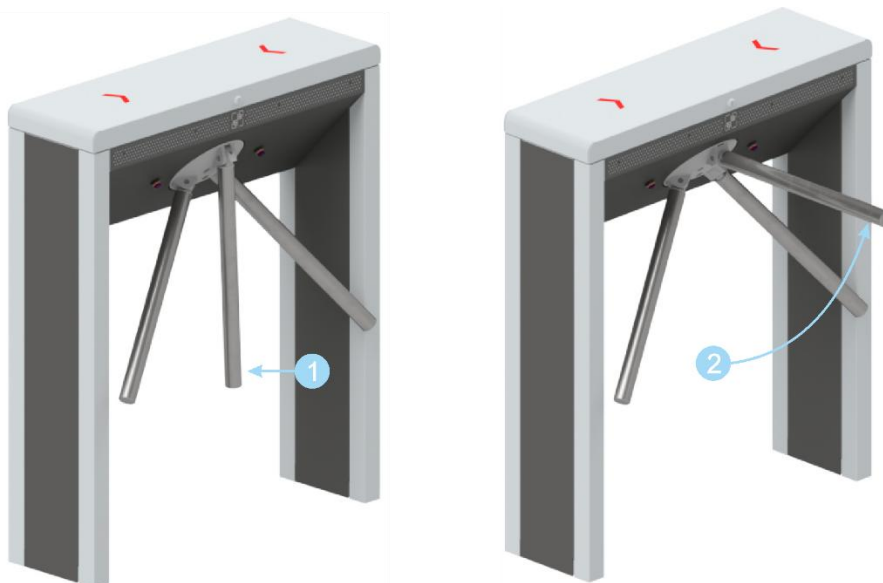
Рисунок 6.5.3 Установка планок в положение блокировки прохода.
