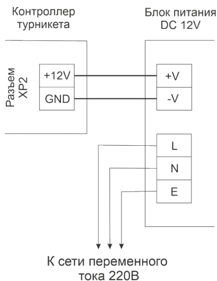
Рисунок 8.4.1 Подключение питания турникета
