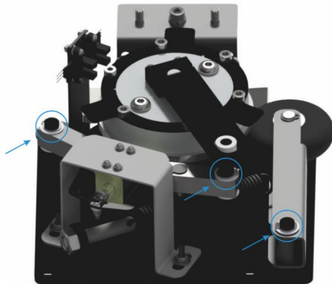
Рисунок 12.5.1 Места смазки подвижных частей
