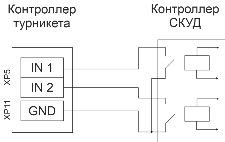
Рисунок 8.2.2 Схема подключения турникета к СКУД «сухой контакт»
