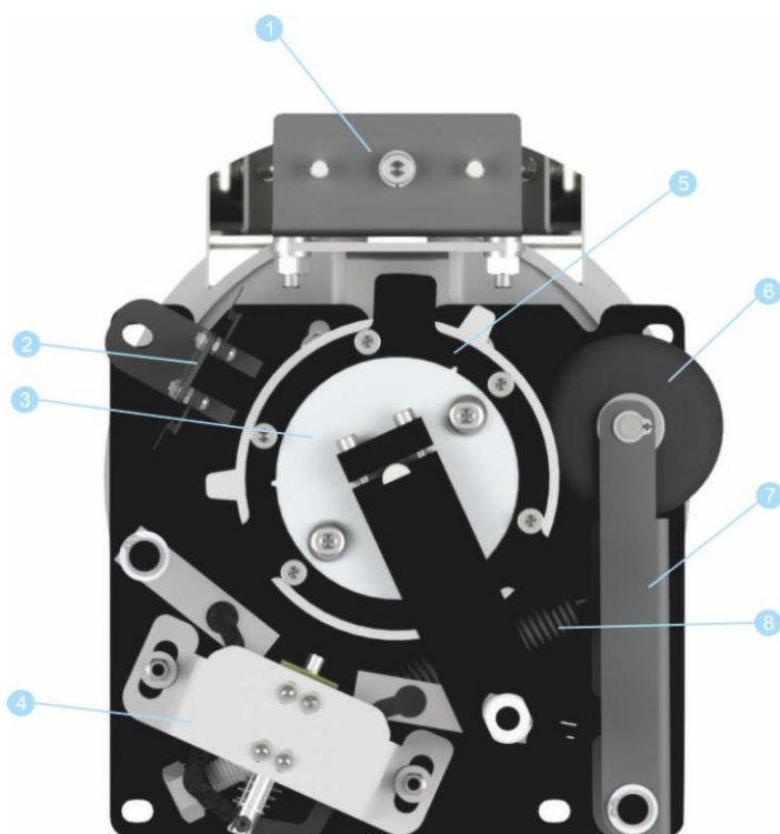
Рисунок 6.2.1. - Устройство механизма турникета
