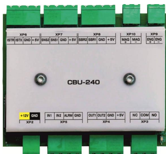
Рисунок 6.3.1 Контроллер управления турникетом «СВU-240»
