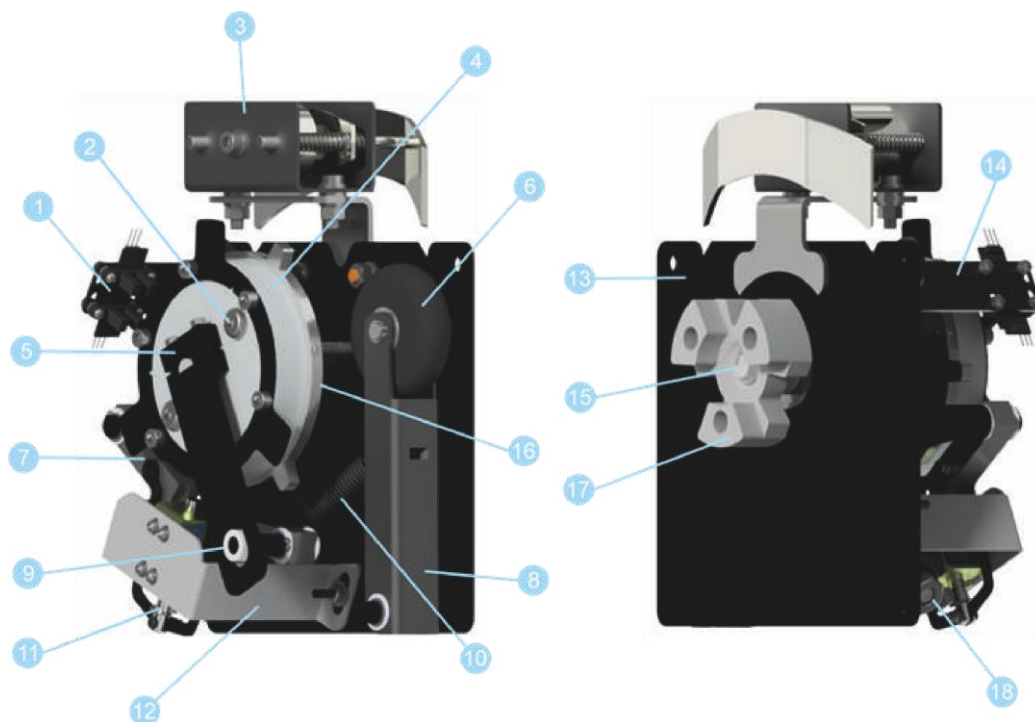
Рисунок 12.2.1 Расположение узлов механизма турникетов
