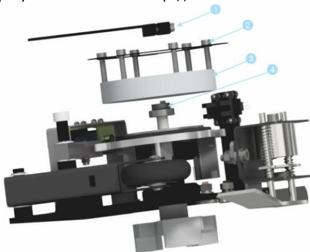
Рисунок 12.3.2 Порядок замены сальника
