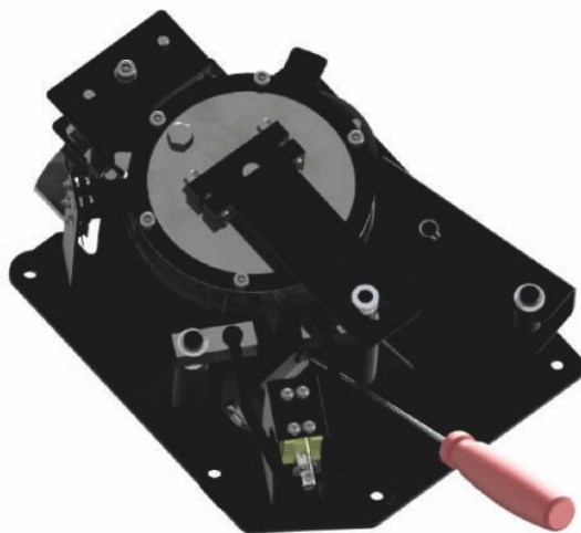
Рисунок 12.4.1 Регулировка натяжения пружины доводчика
