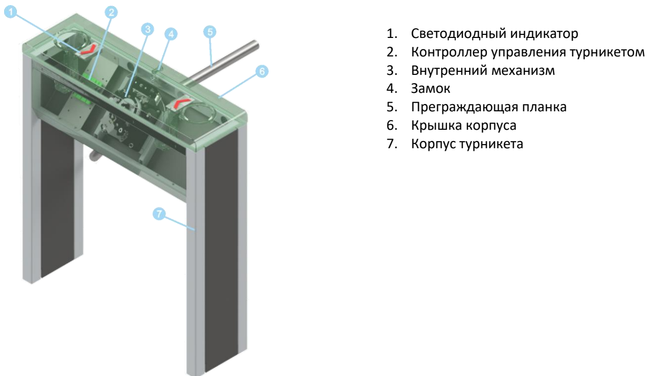
Рисунок 6.1. - Внешний вид турникета
