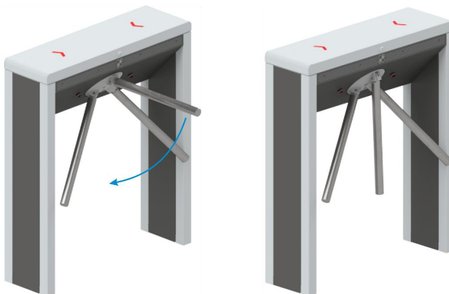
6.5.2 Принцип работы автоматической системы разблокировки прохода
