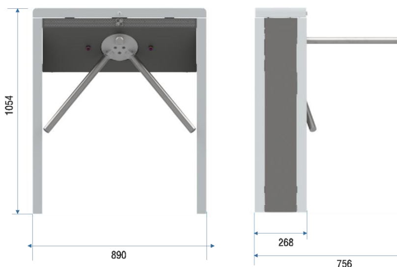
Рисунок 5.1 Габаритные размеры турникета
