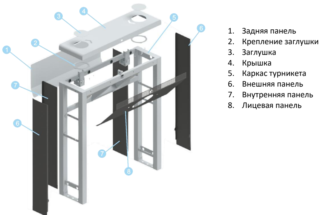
Рисунок 6.11. - Внешний вид турникета
