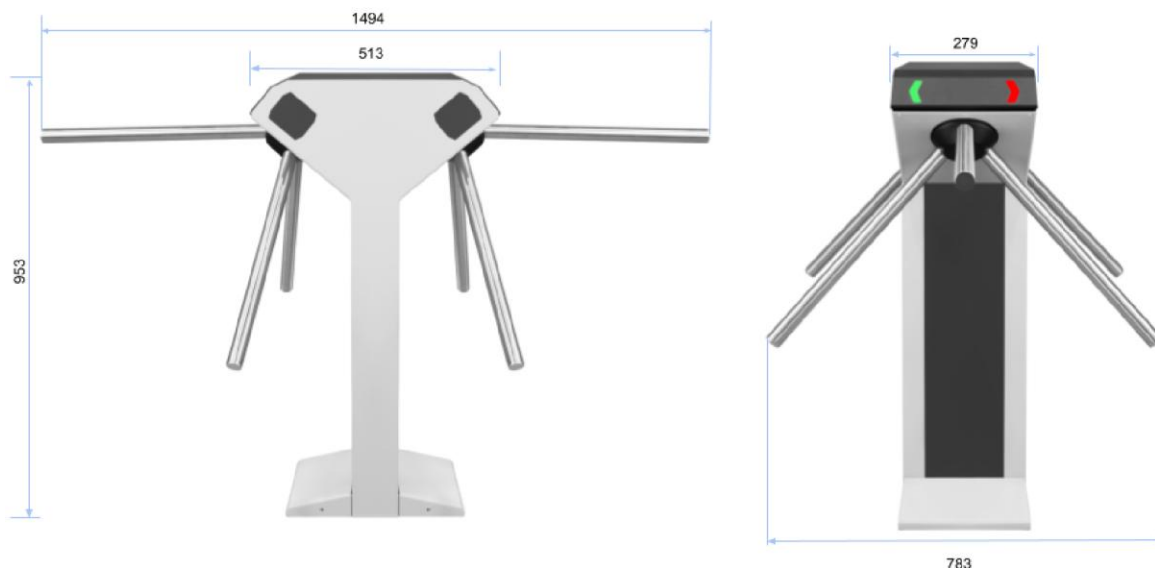
Рисунок 5.1 - Габаритные размеры турникета с планками
