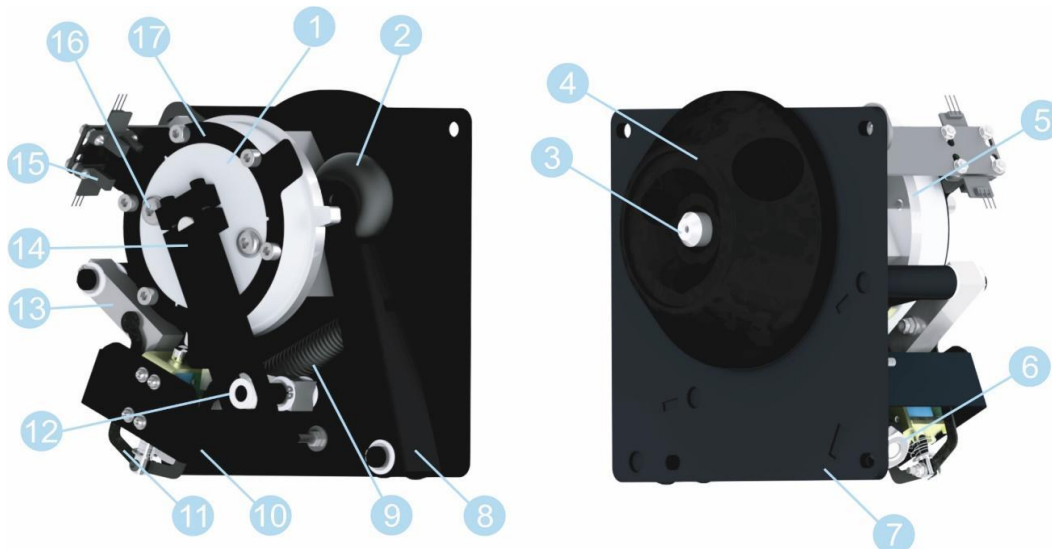
Рисунок 12.2.1 - Расположение узлов механизма турникета ТМ-1
