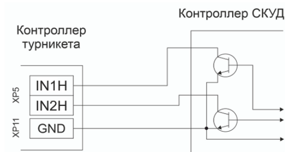
Рисунок 8.2.3 Схема подключения турникета к СКУД «открытый коллектор»
