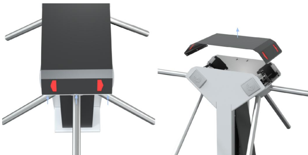
Рисунок 12.1.1 - Демонтаж верхней крышки турникета
