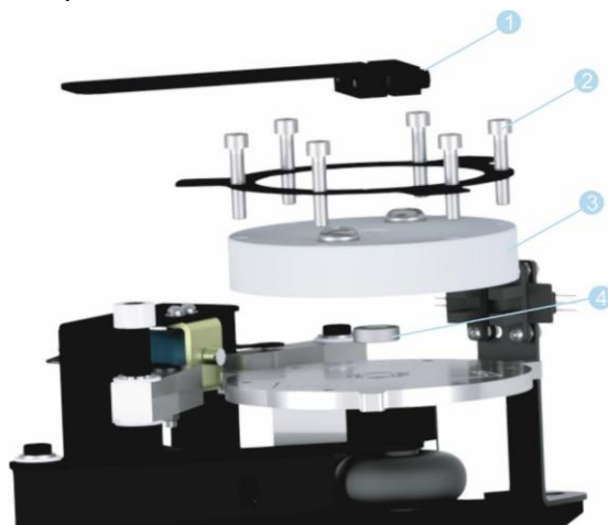
Рисунок 12.3.2 - Порядок замены сальника
