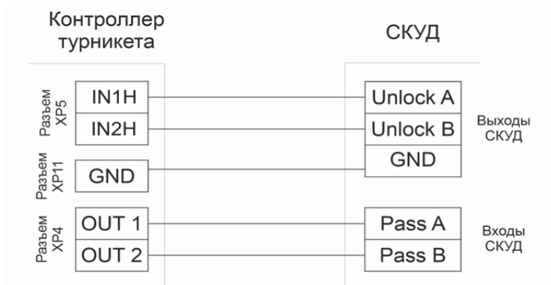
Рисунок 8.2.1 - Подключение турникета к стороннему СКУД
