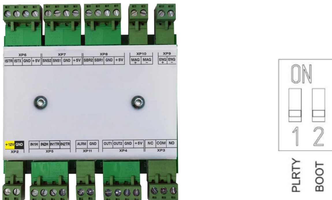
Рисунок 6.3.1 Контроллер управления турникетом «СВU-240» Dip-переключатели
