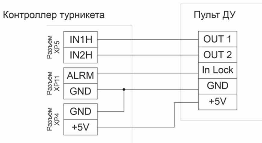
Рисунок 8.1.1. Схема подключения пульта управления
