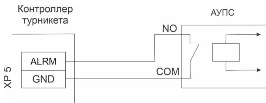
Рисунок 8.3.1 - Подключение АПС к турникету
