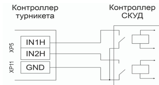
Рисунок 8.2.2 Схема подключения турникета к СКУД «сухой контакт»
