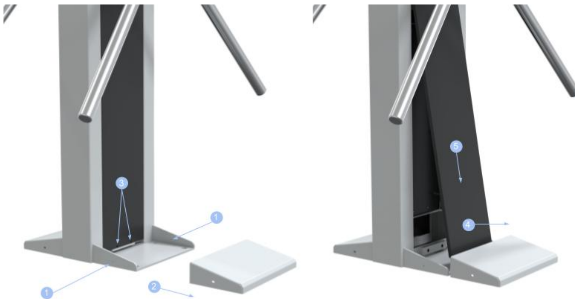
Рисунок 7.4.2 - Разборка кожухов турникета
