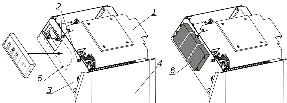
Рисунок 13. Вид турникета без крышки, места установки считывателей
