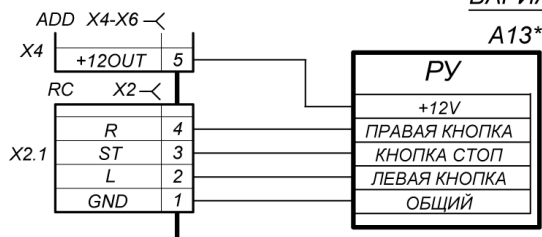
Рисунок 20. Схема электрическая соединений
