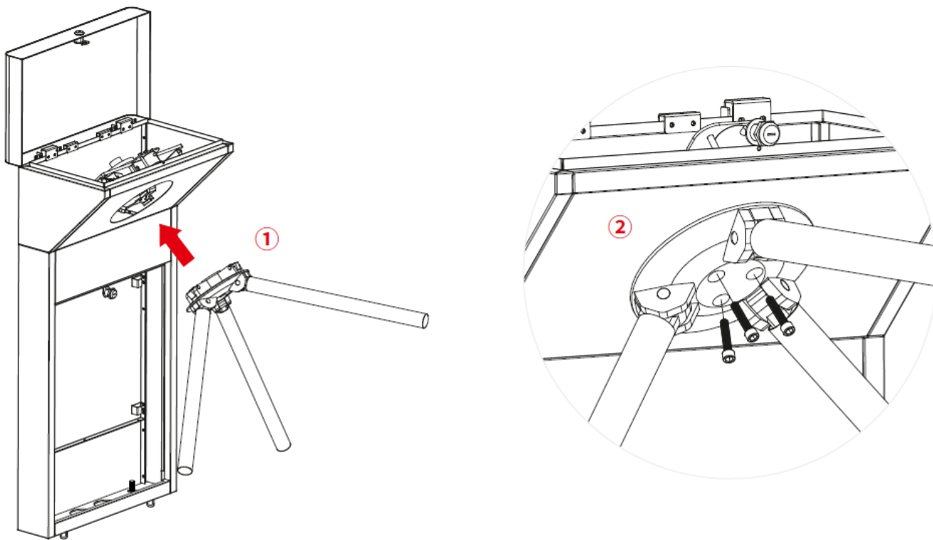
Рисунок 6. Установка блока планок
