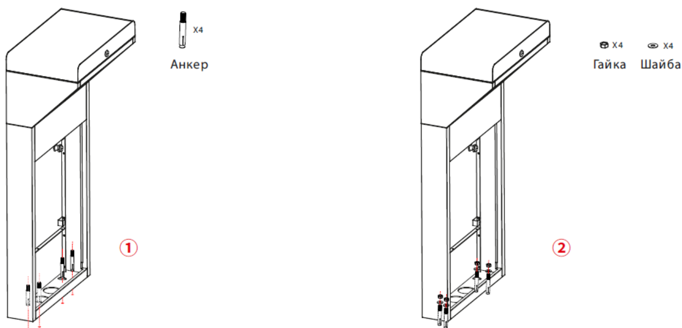
Рисунок 5. Крепление турникета
