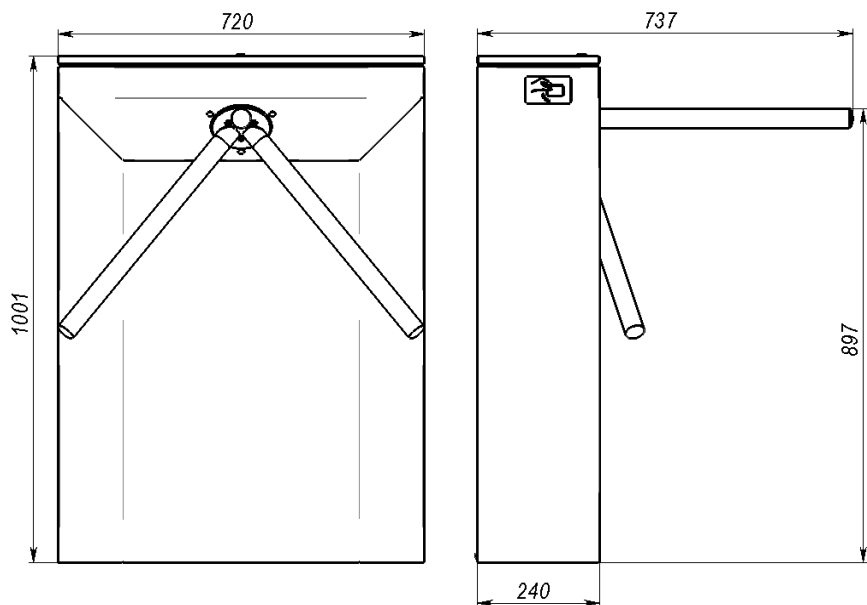
Рис.7Б3 Турникет SA400 (SA401). Габаритные размеры
