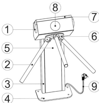
Рисунок 1 Внешний вид и элементы подключения
