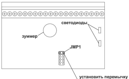
Рисунок 3 Контроллер СКУД
