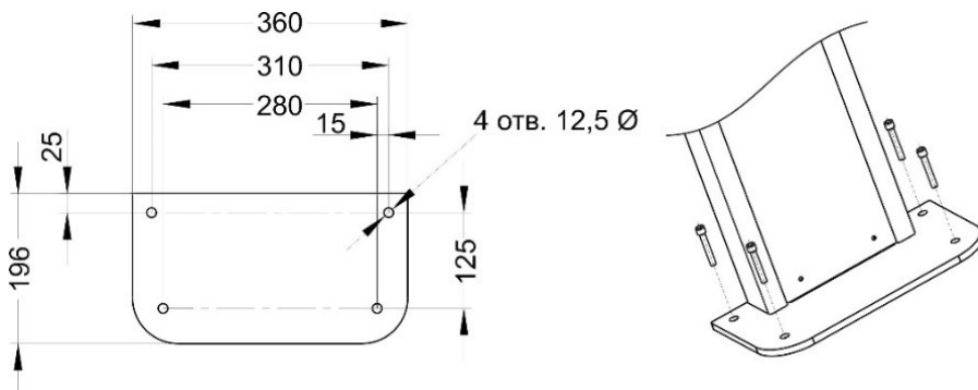
Рисунок 5 Установка проходной на основание
