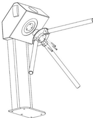
Рисунок 6 Установка ступицы со штангами ограничителями.
