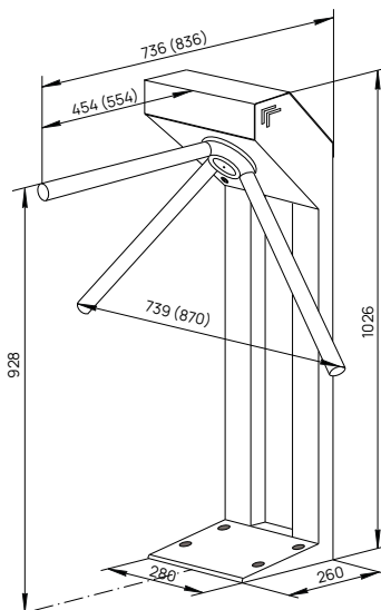
Габаритные размеры
