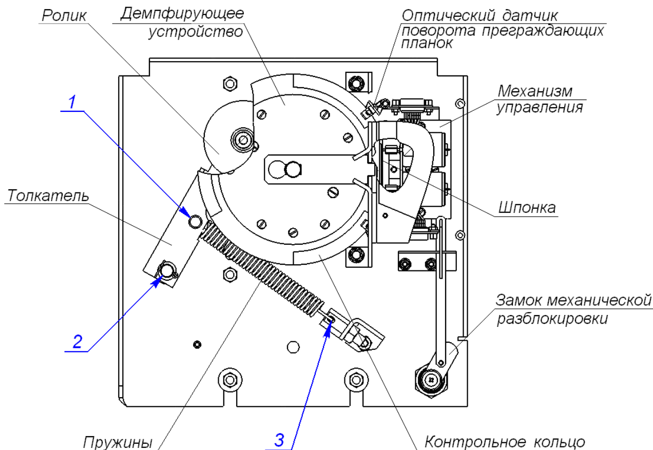
1, 2, 3 - места смазки
