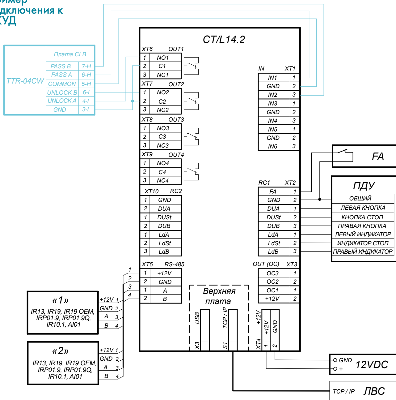
Пример схемы подключения турникета к контроллеру СКУД
