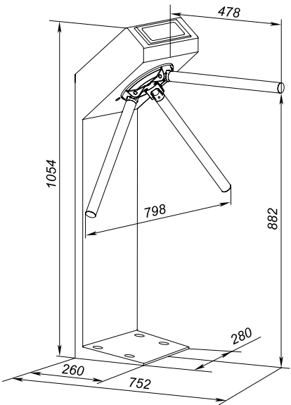
Габаритные размеры
