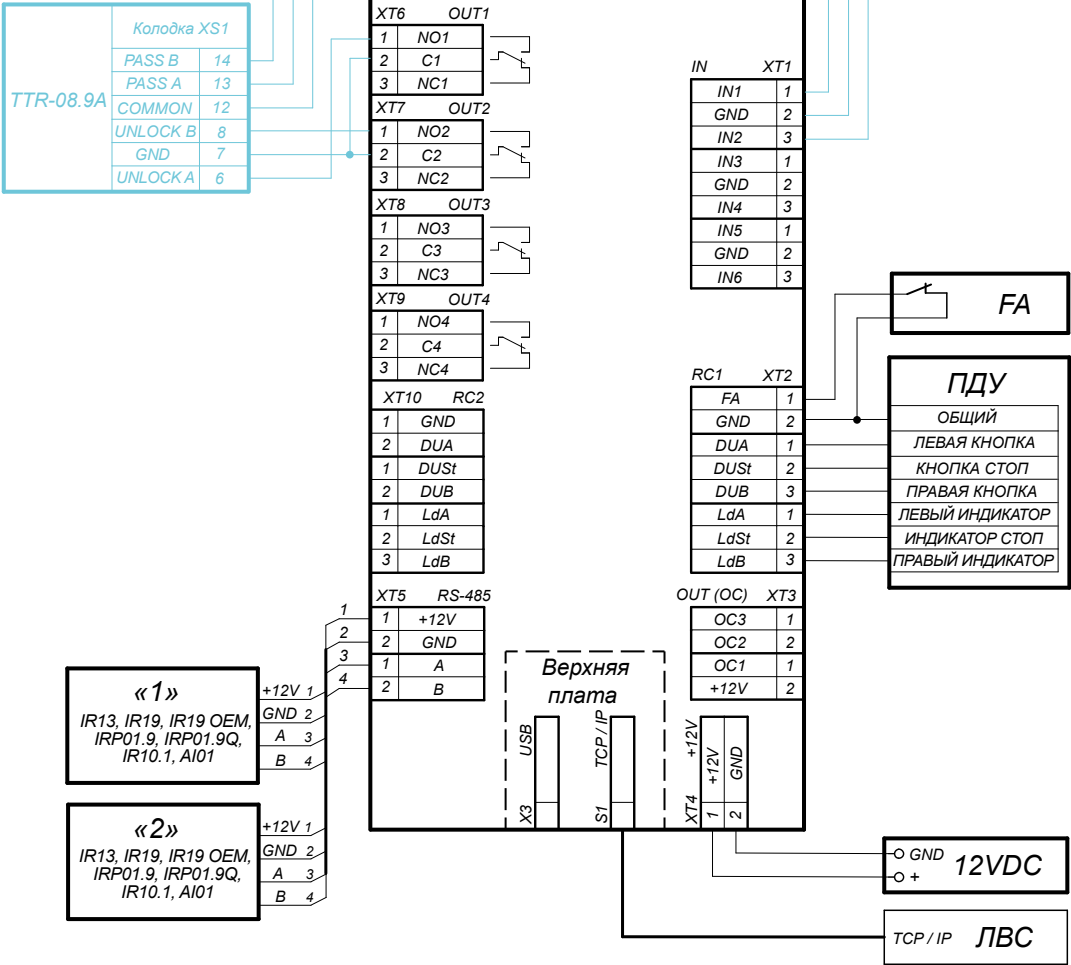
Пример схемы подключения турникета к контроллеру СКУД
