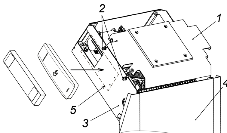
Рисунок 13. Вид турникета без крышки, места установки считывателей
