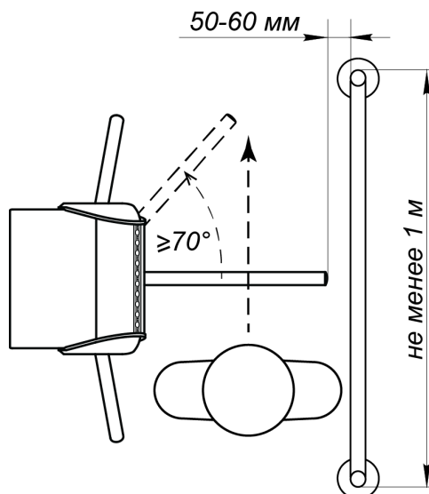
Рисунок 9. Рекомендации по организации зоны прохода
