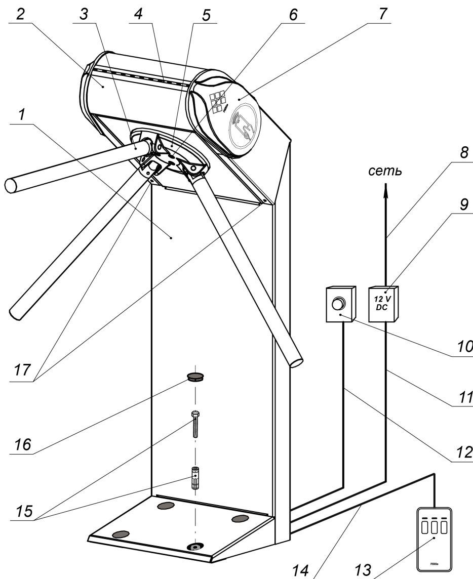
Рисунок 2. Общий вид турникета
