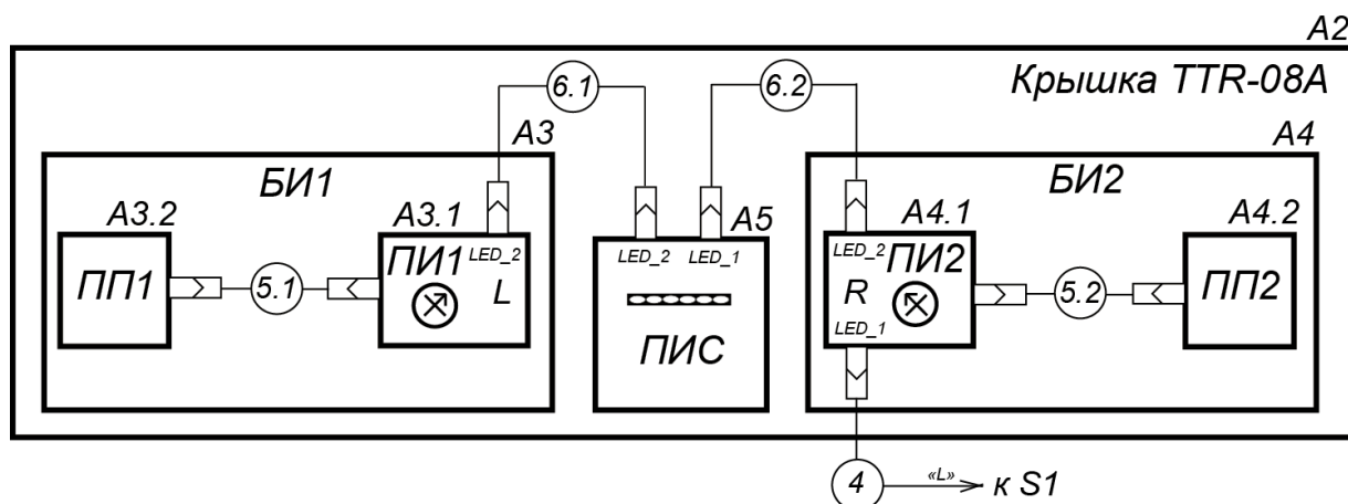
Рисунок 10. Схема электрическая соединений крышки турникета (A2)
