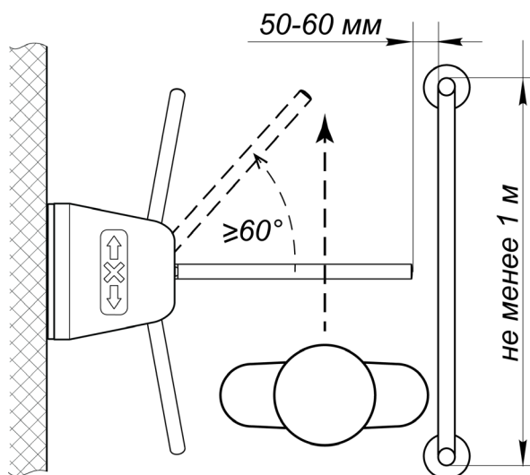
Рисунок 16. Рекомендации по организации зоны прохода
