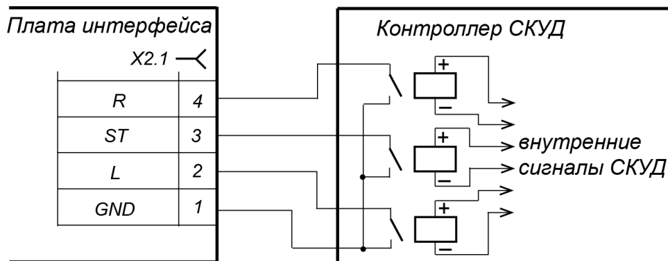
Рисунок 11. Управляющий элемент СКУД – нормально разомкнутый контакт реле
