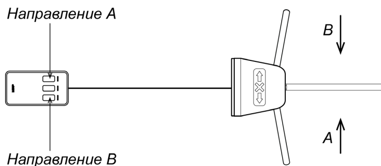
Рисунок 13. Стандартная ориентация ПДУ относительно стойки турникета
