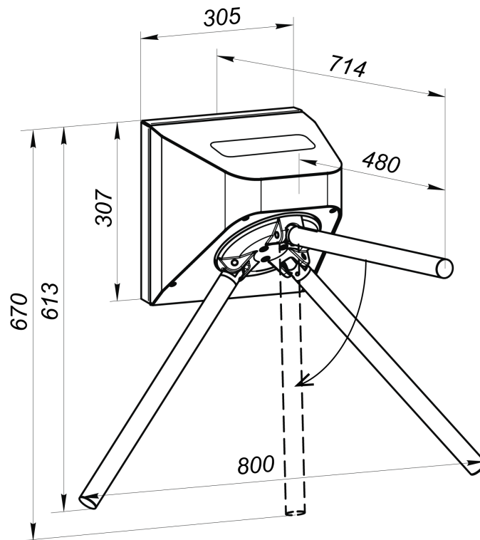
Рисунок 3. Габаритные размеры PERCo-TTR-10AK
