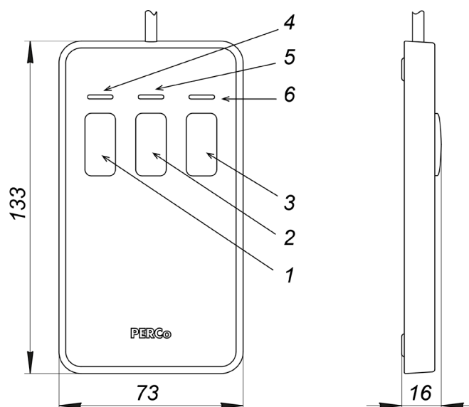
Рисунок 8. Общий вид и габаритные размеры ПДУ
