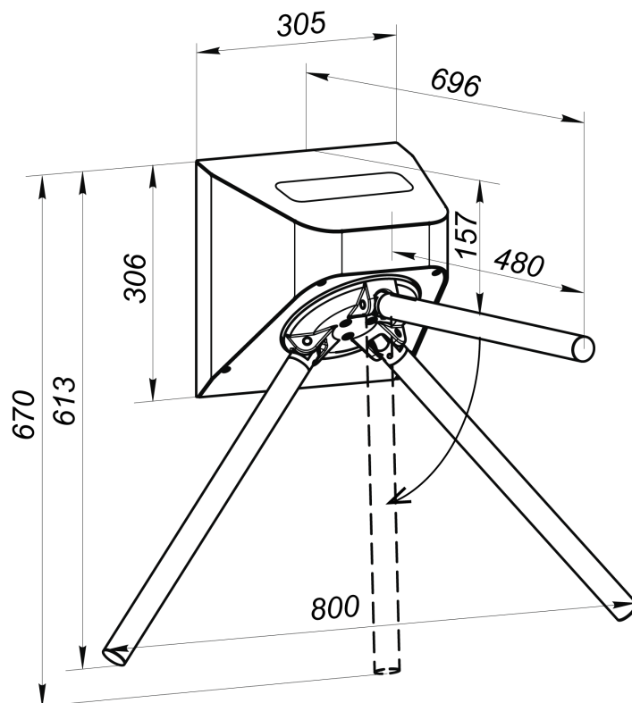
Рисунок 1. Габаритные размеры турникета без монтажного кронштейна (стойки)
