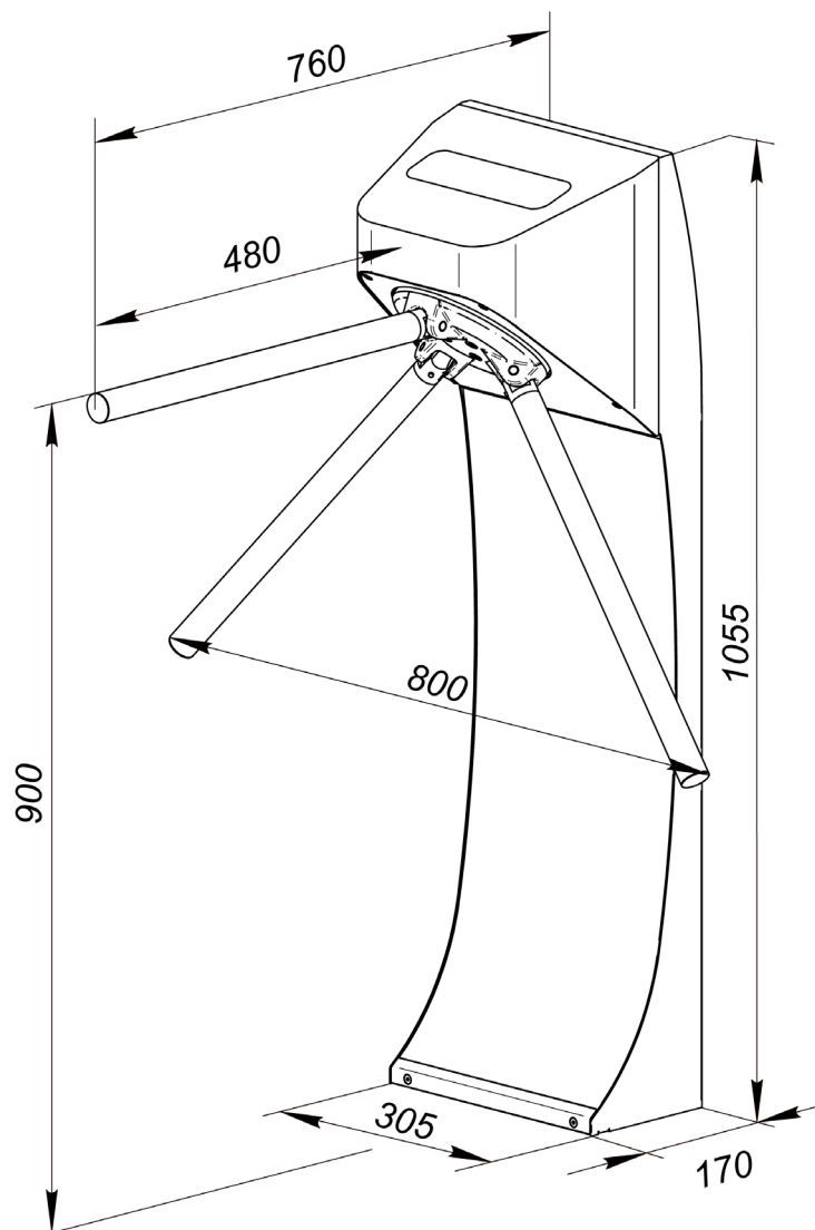
Рисунок 4. Габаритные размеры PERCo-TTR-10AB
