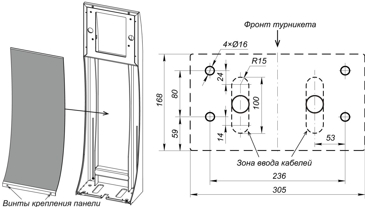
Рисунок 19. Порядок монтажа и схема разметки отверстий для стойки PERCo-MT10.3¹
