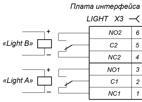
Рисунок 12. Выходные каскады для Light A и Light B
