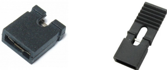
Рисунок 4.2 – Джамперы (перемычки)
