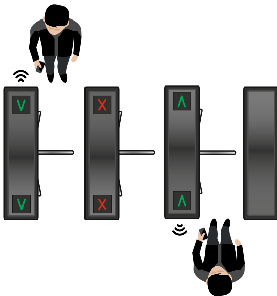
Рисунок 11.1 - Использование формирователя прохода без переноса табло и считывателей
