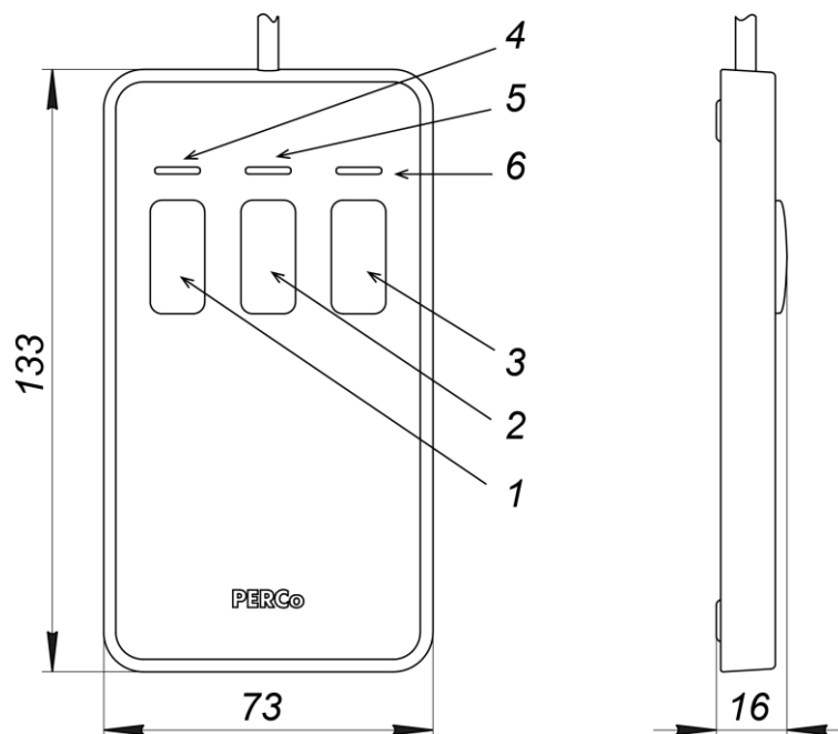
Рисунок 3. Общий вид и габаритные размеры ПДУ
