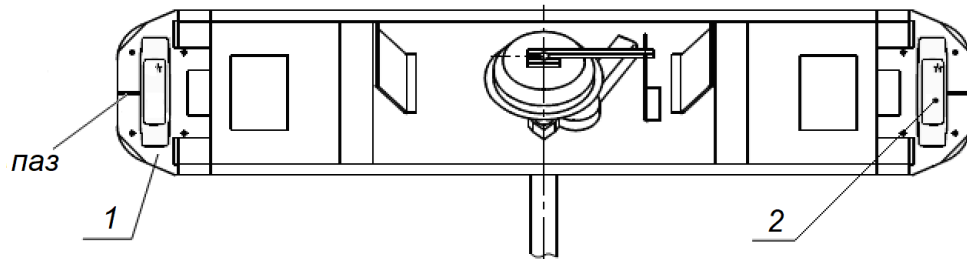
Крышка турникета (вид снизу)
