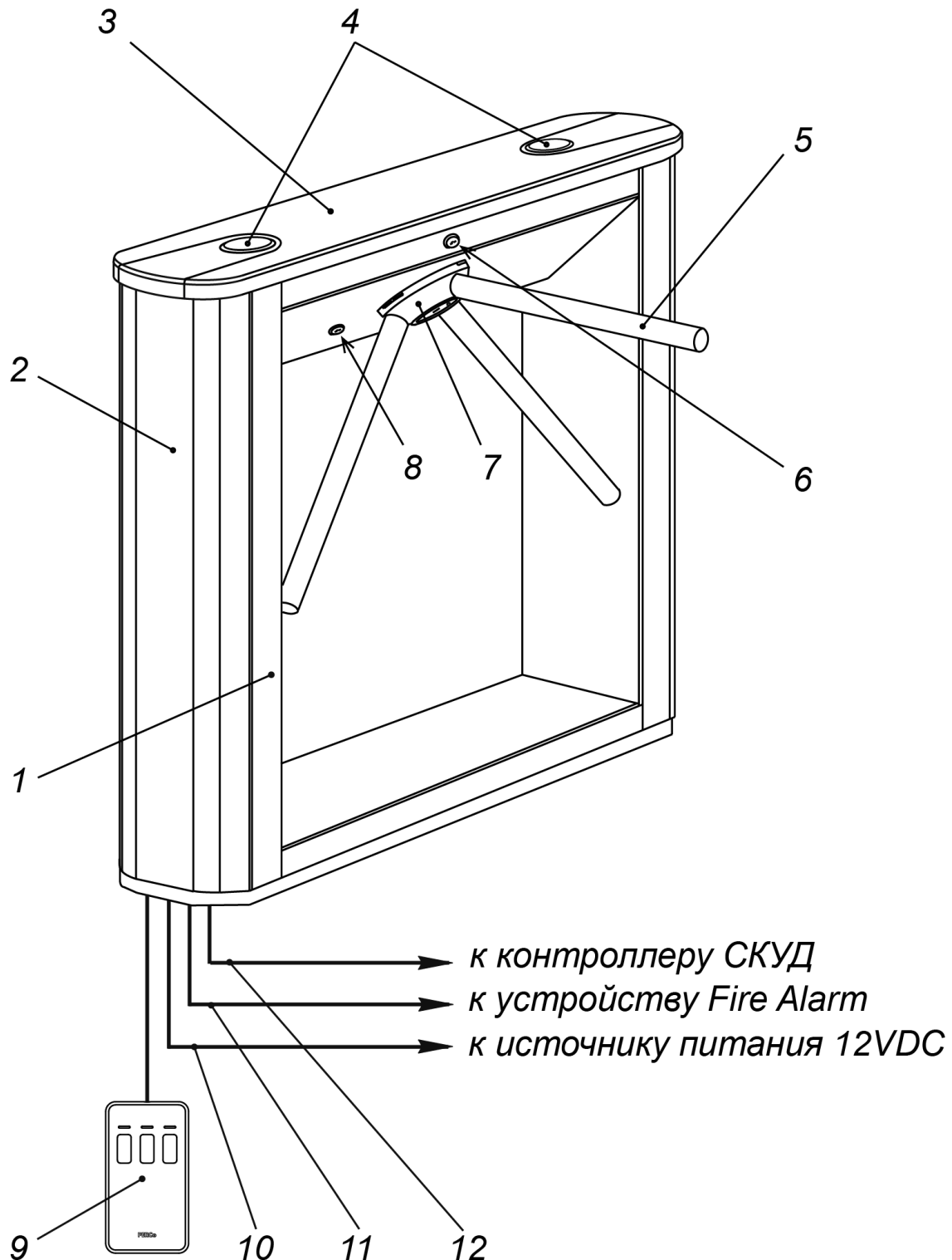
Рисунок 2. Общий вид турникета
