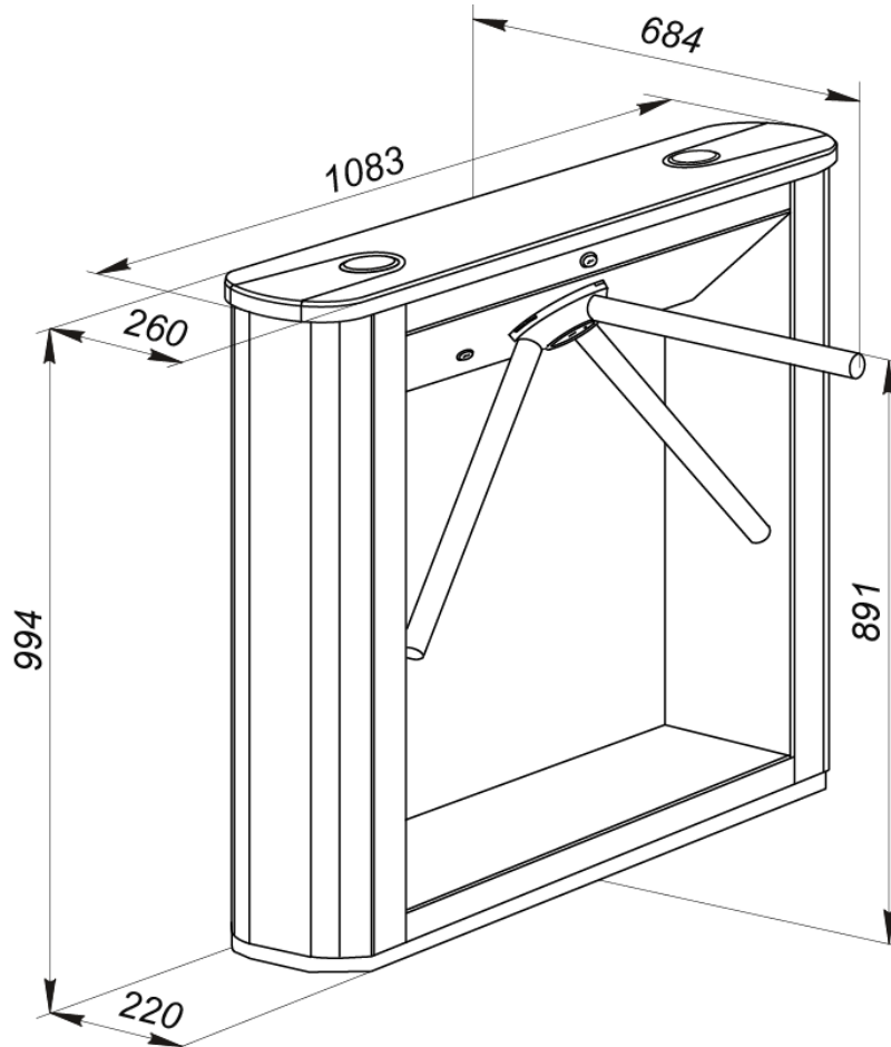
Рисунок 1. Габаритные размеры турникета
