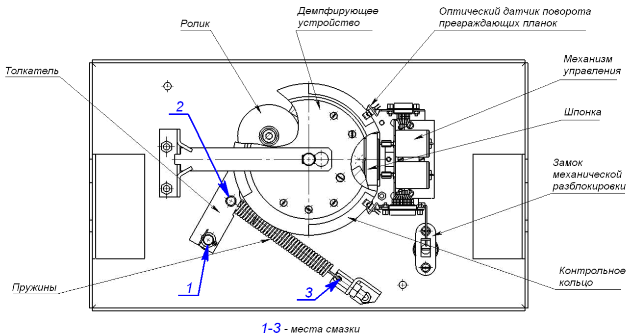
Рисунок 15. Расположение внутренних деталей и узлов стойки турникета
