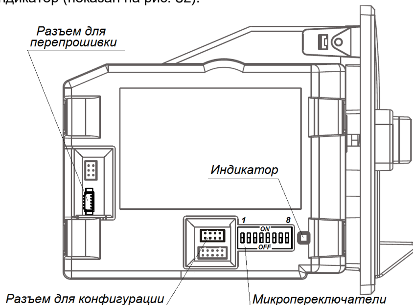
Рисунок 32. Расположение разъемов
