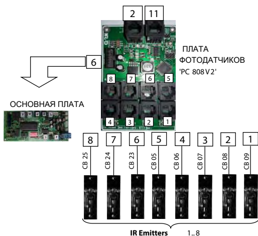
Модуль приемника
