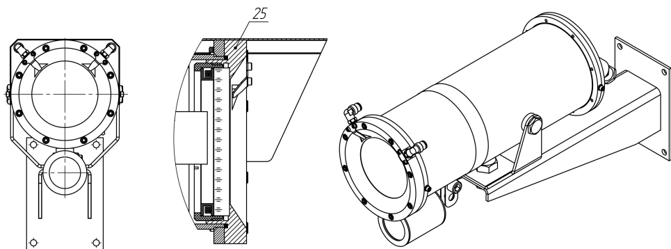
Рисунок 6. Внешний вид термокожуха TBK-07-O-H/C с установленным фланцем (СОД) для работы с системой очистки стекла “Дуплекс-07е”-Ех-TBK-X.
