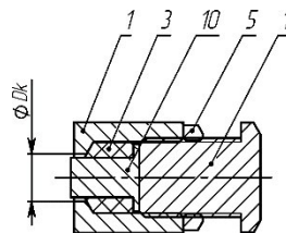
ж) монтаж заглушки 3Г
