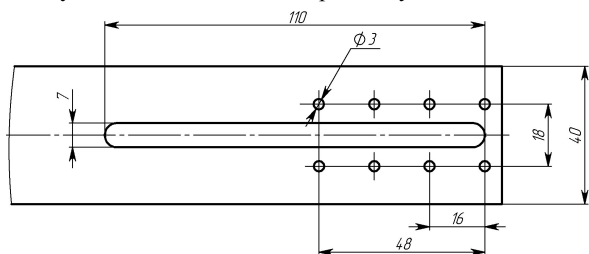
Рисунок 3. Внешний вид термокожуха ТВК-07-О-В.
