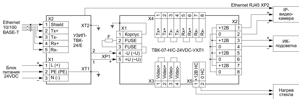
Рисунок 15. Примеры подключения термокожухов
