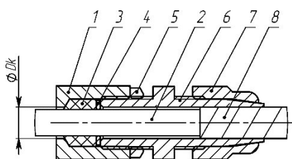
а) монтаж бронированным кабелем в кабельном вводе КВ512
