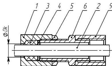
б) монтаж в трубной разводке с помощью штупера ШТ
