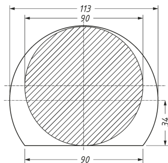
а) TBK-07-O-H/C: Ø113x240 мм (DxL)
