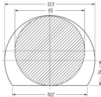
б) TBK-07-O-B: Ø123x240 мм (DxL)
