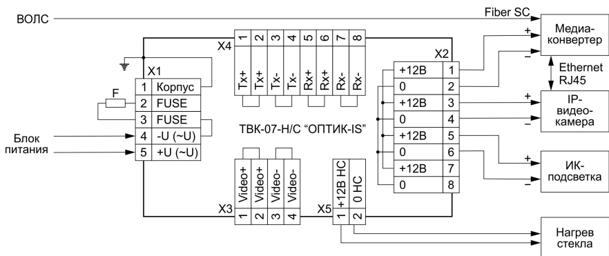
б) Подключение термокожуха на примере модификации TBK-07-О-Н-“ОПТИК-IS”-УХЛ1 с ИК-подсветкой, IP-видеокамерой и медиаконвертером
