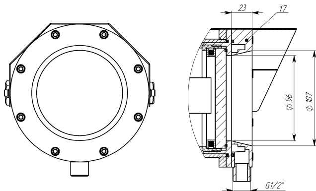
Рисунок 5. Установка бленды (БЗП) на примере термокожуха TBK-07-O-H/C.
