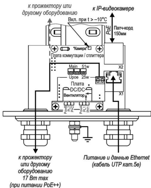
Рисунок 7 – Схема подключения TBK-...-PoE++
