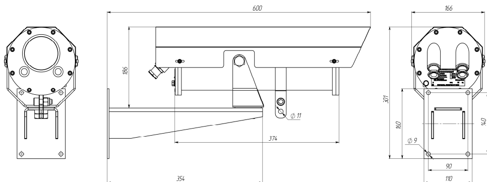
Рисунок 3. Внешний вид видеокамер ТВК-БК-07-3XX-H(C)400 со встроенным модулем ИК-подсветки (IRF, опция).
