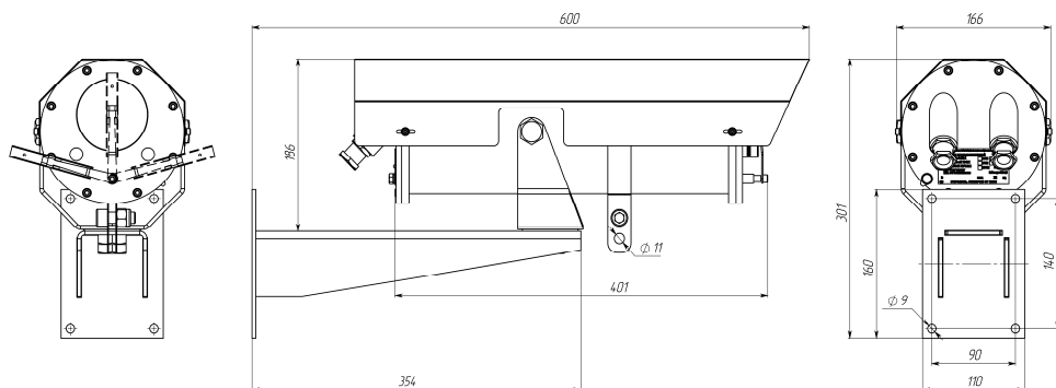
Рисунок 4. Внешний вид видеокамер ТВК-БК-07-3XX-H(C)400 со встроенным модулем ИК-подсветки (IRF, опция) и очисткой стекла (W, опция).
