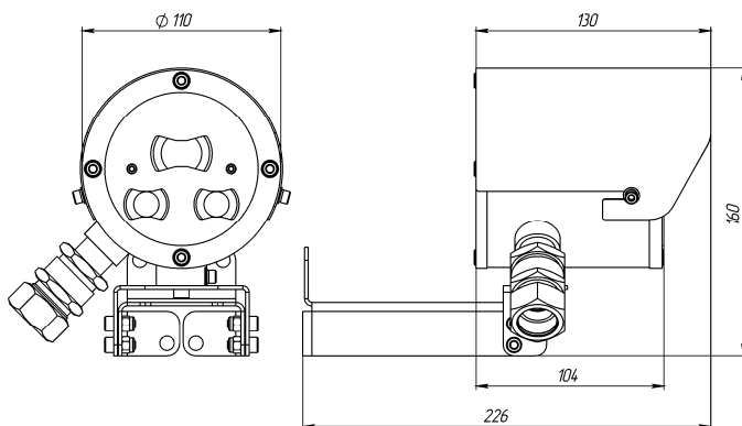
Рисунок 1. Внешний вид видеокамеры ТВК-БК-07-2XX-H100.
