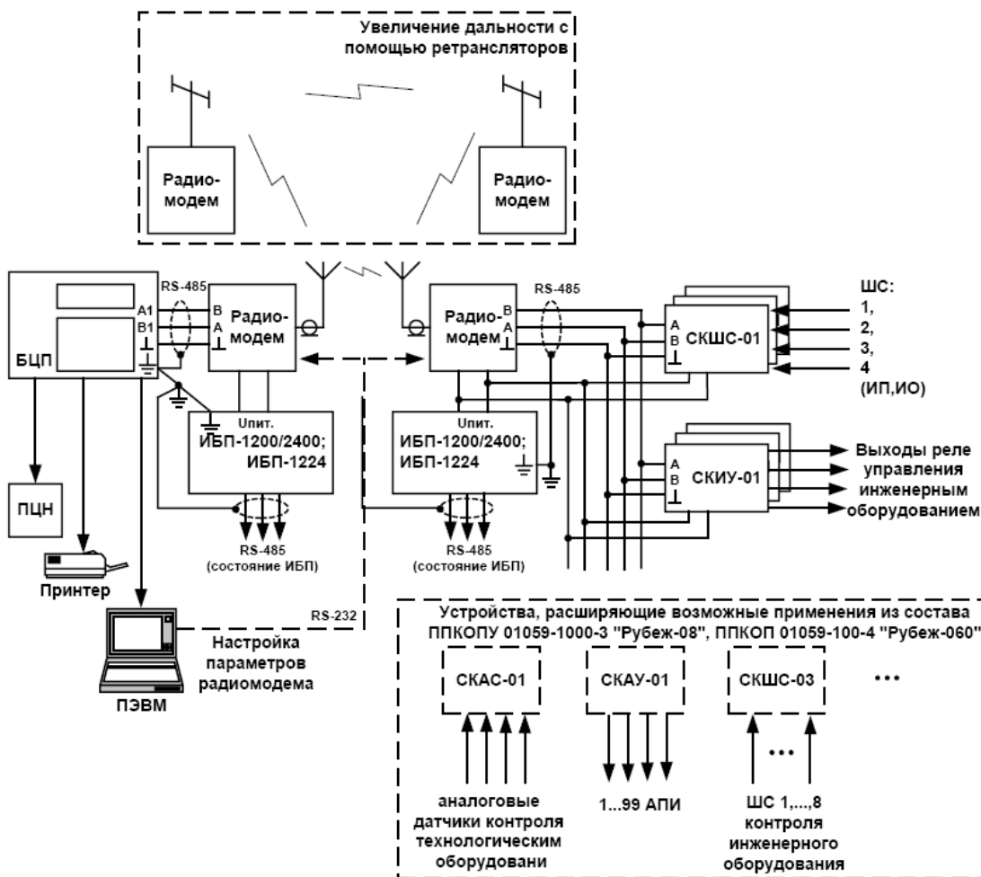
Рисунок 14 Структура ИСБ на основе аппаратуры «Рубеж» с передачей данных по радиоканалу
