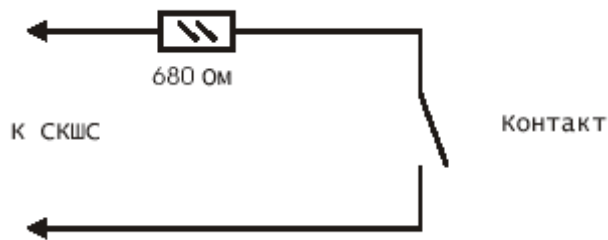
Рисунок 45 Схема включения ШС с контролем КЗ
