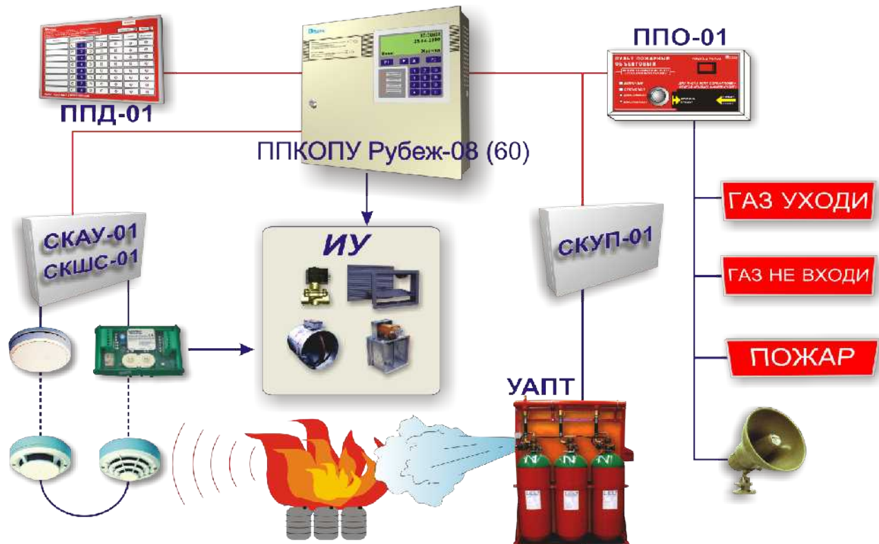
Рисунок 108 Структурная схема построения системы пожарной сигнализации, автоматического пожаротушения и управления противопожарной автоматикой на основе ИСБ «Рубеж-08»
