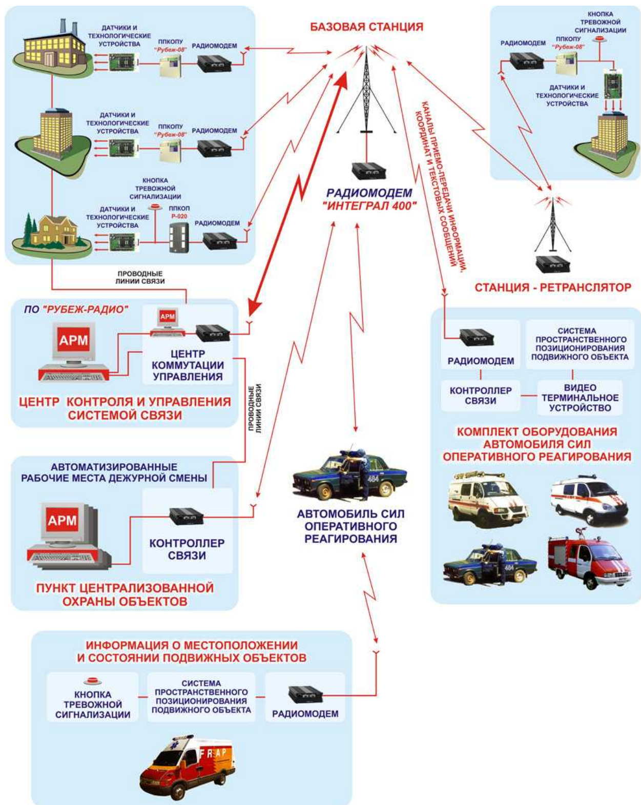
Рисунок 112 Структурная схема системы информационно-телекоммуникационного обеспечения оперативных служб на базе радиомодема «Интеграл-400»
