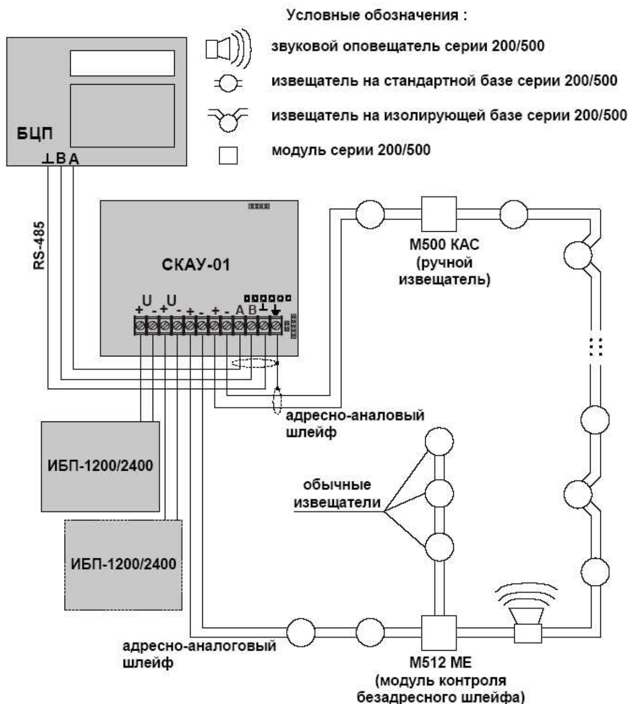
Рисунок 71 Типовая схема включения СКАУ-01
