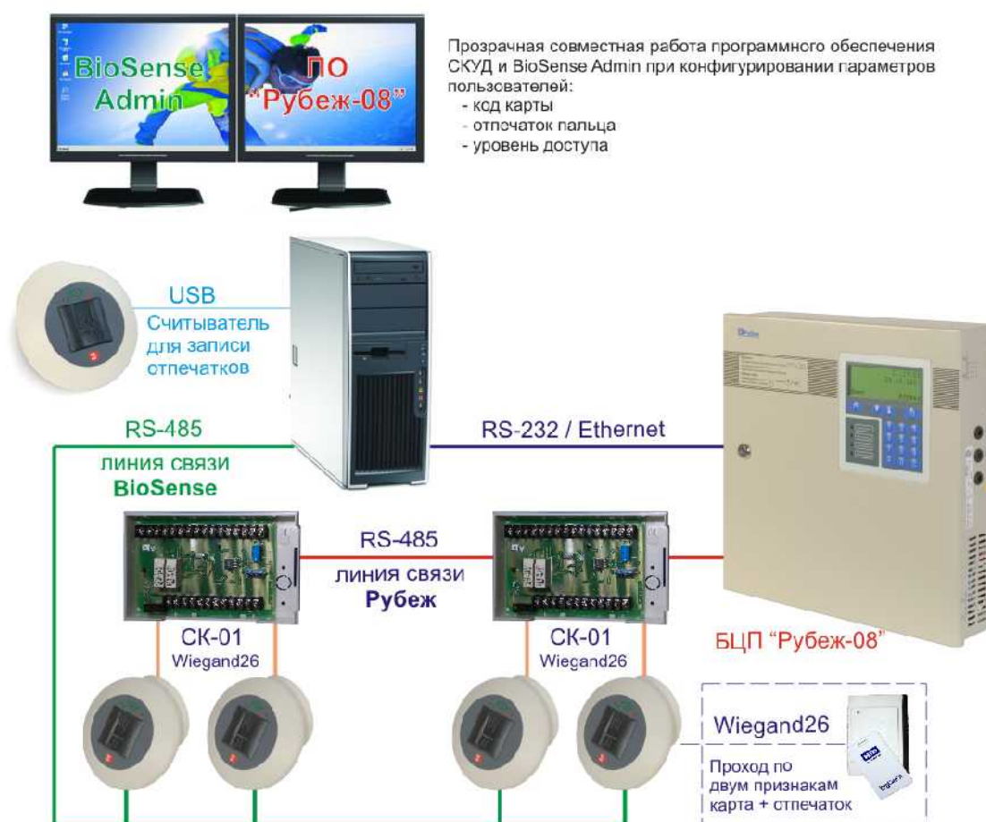
Рисунок 81 Варианты применения биометрического считывателя
