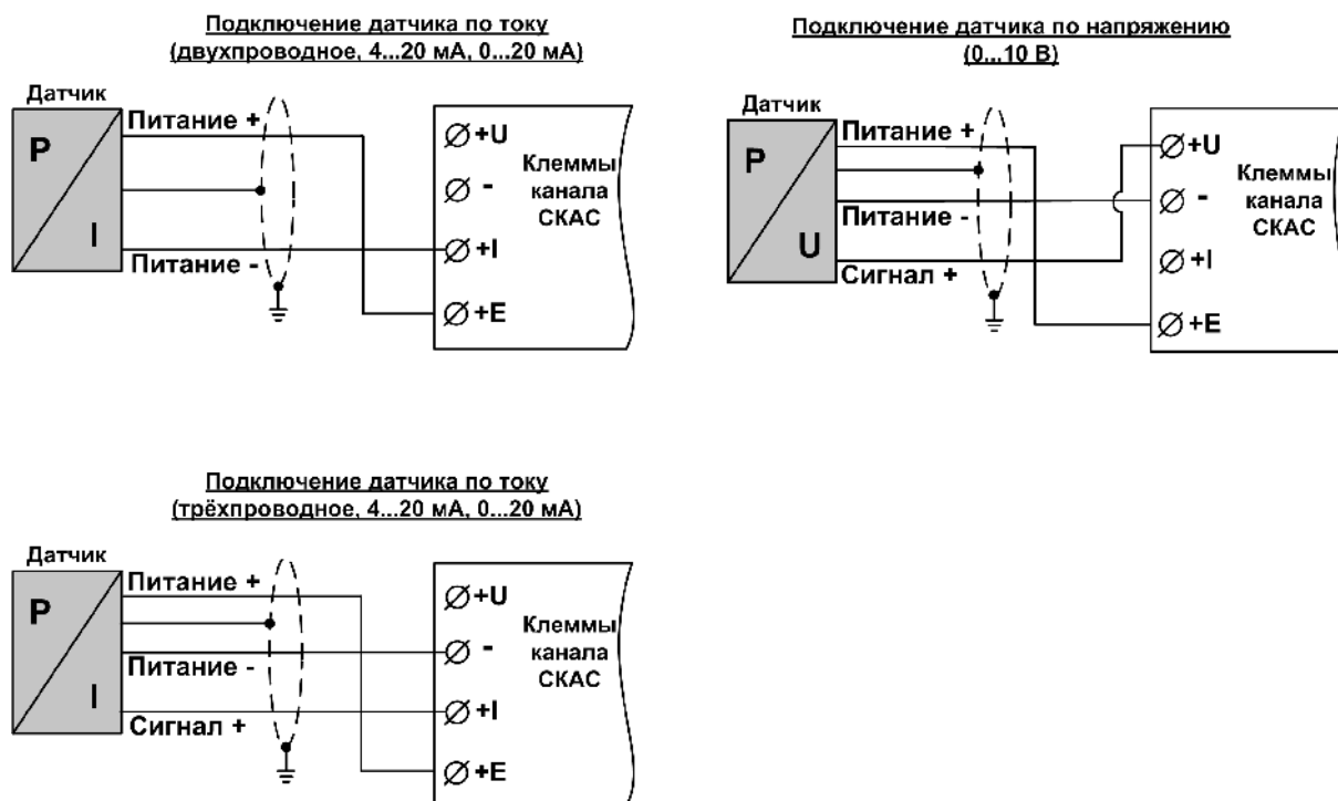
Рисунок 49 Примеры подключения датчиков с питанием от SKAS
