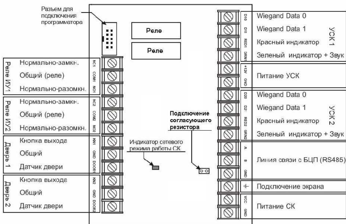
Рисунок 74 Подключение внешних цепей и устройств к контроллеру доступа СК-01
