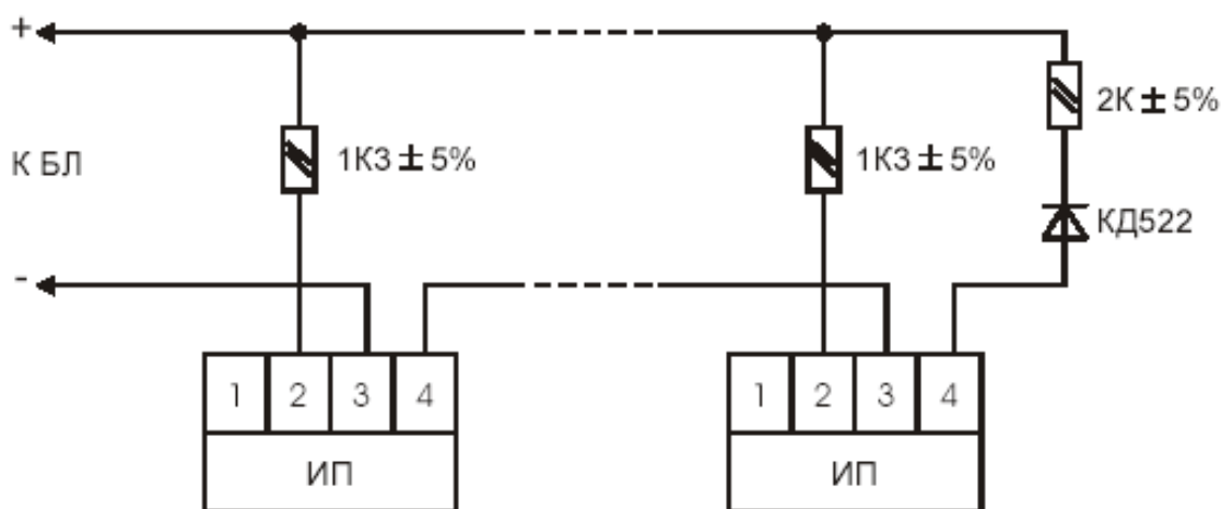
Рисунок 56 Схема включения ИП с нормально-разомкнутыми контактами (ИП-212-5М и т.п.) в ШС типа 4, 6
