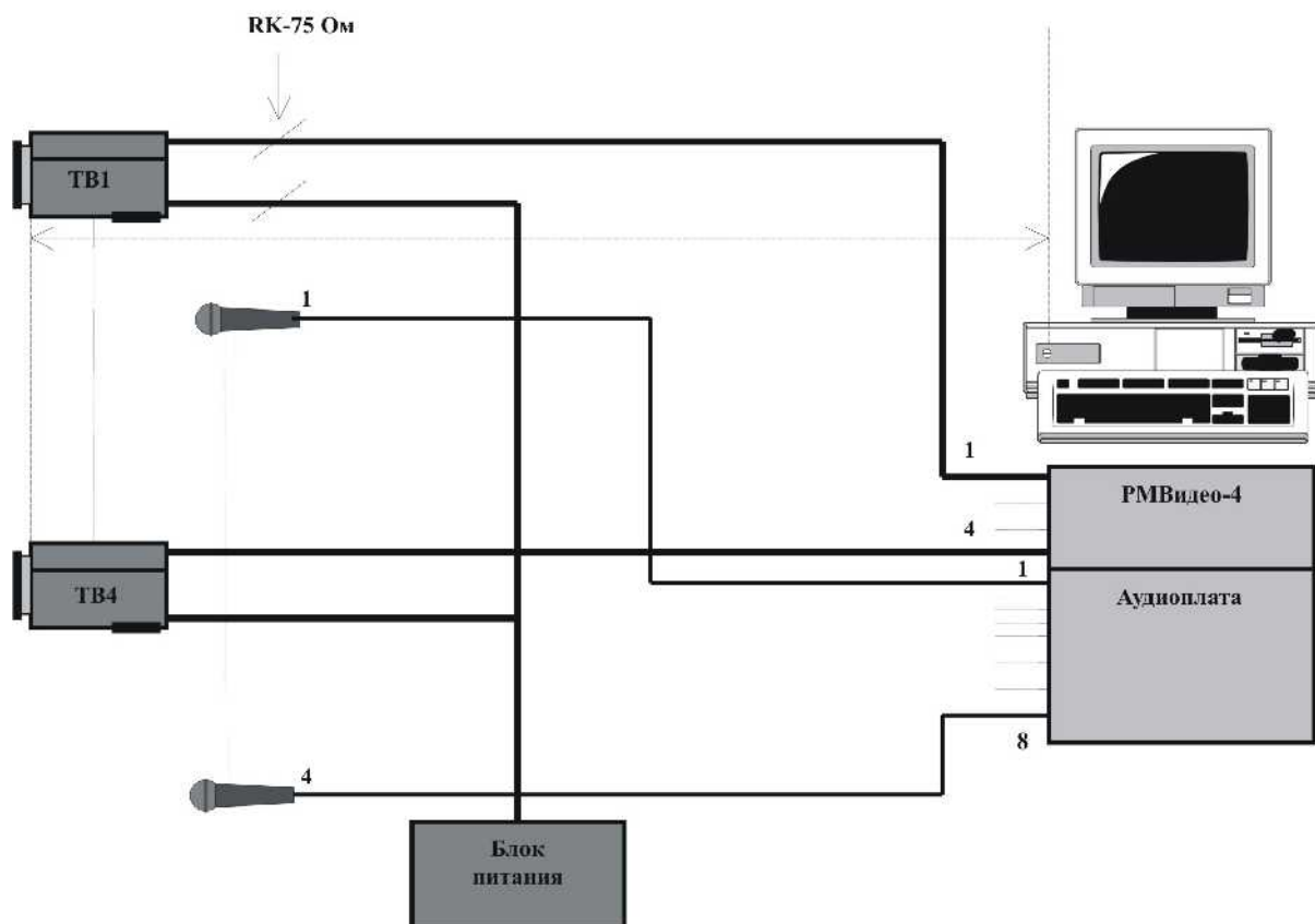
Рисунок 84 Конфигурация системы с одним компьютером
