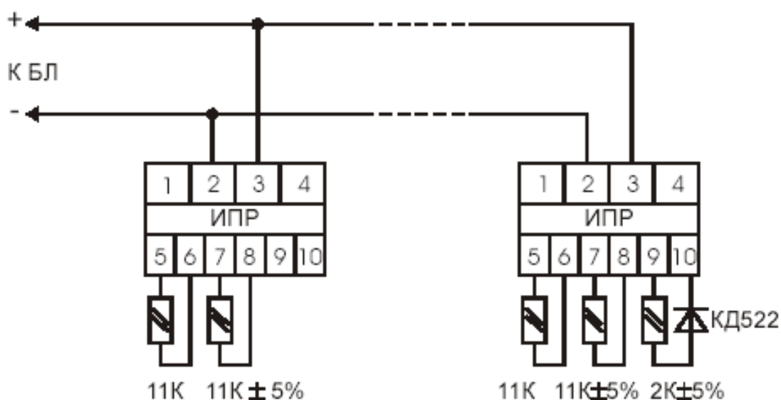
Рисунок 57 Схема включения ручного ИП (ИПР и т.п.) в ШС типа 4, 6
