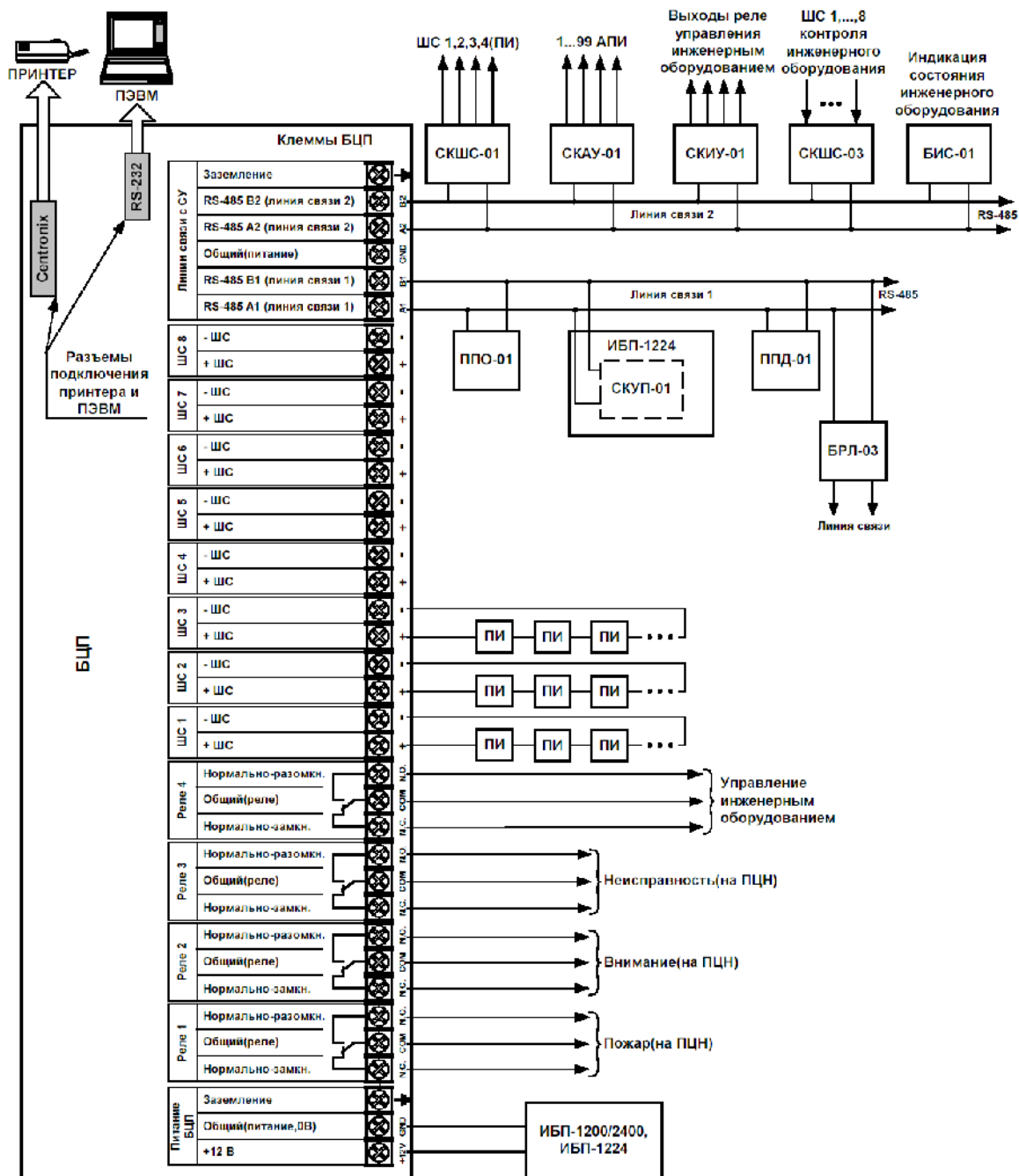
Рисунок 110 Подключение дополнительных устройств для расширения возможностей АСПТ
