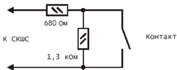
Рисунок 44 Типовая схема включения ШС с контролем КЗ и обрыва
