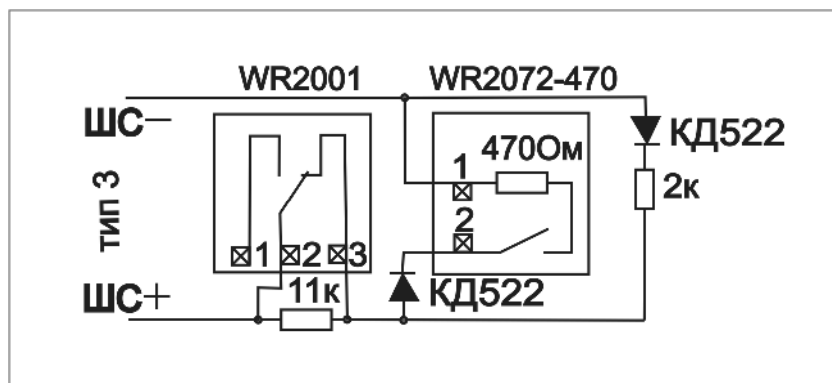
Рисунок 63 Последовательное включение ручных пожарных извещателей WR2000 (тип шлейфа 3)
