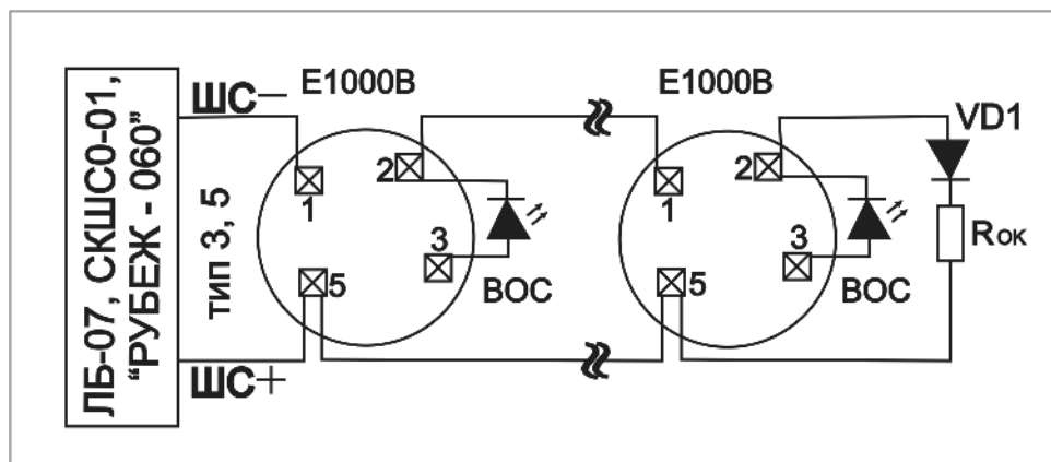
Рисунок 62 Подключение извещателей серии ЕСО1000 при формировании извещения «Пожар» по одному датчику (тип шлейфа 3 или 5).
