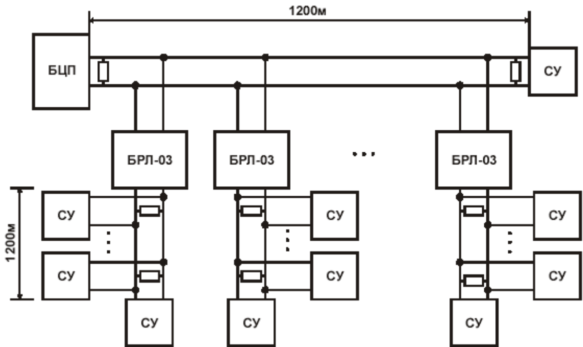
Рисунок 5 Применение БРЛ для ветвления линии с связи
