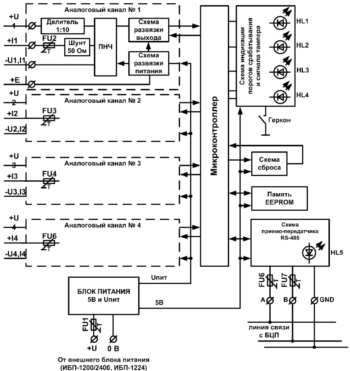
Рисунок 48 Структурная схема SKAS
