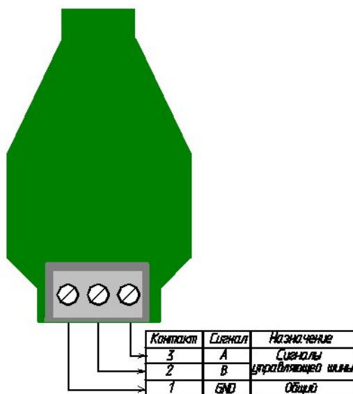
Рисунок 2 - Схема подключения устройства
